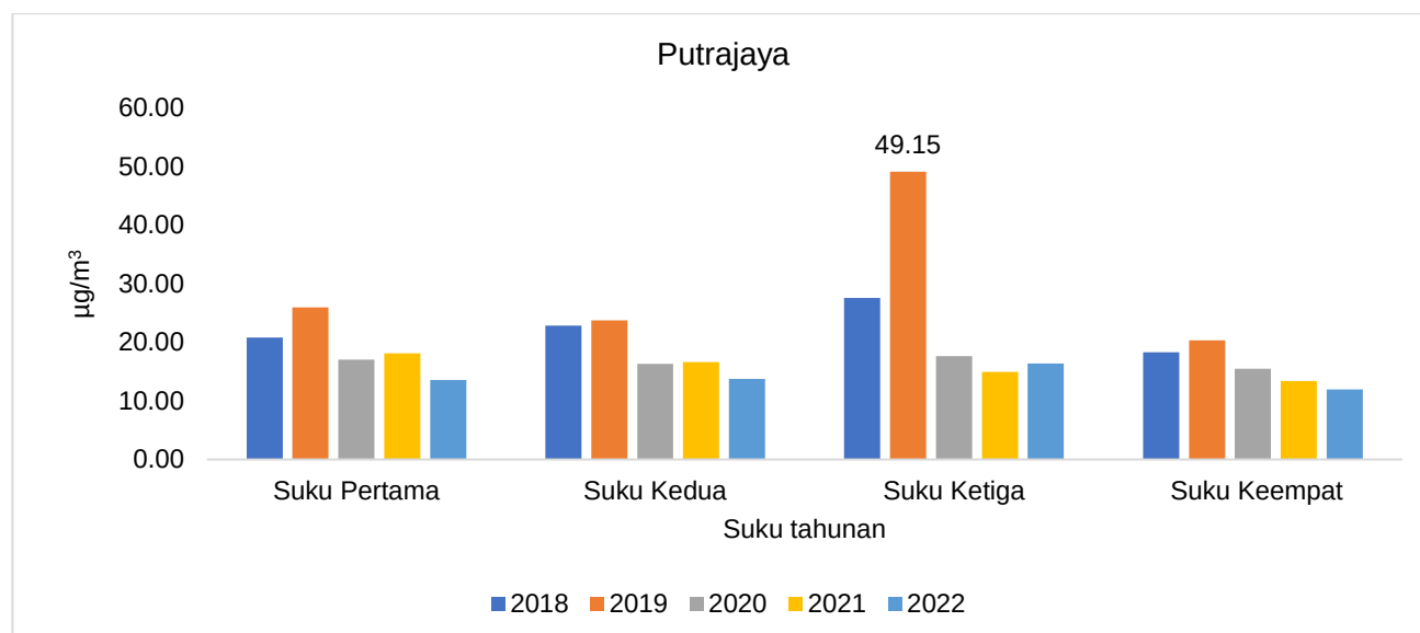
Carta 1.4: Purata suku tahunan kepekatan Habuk Halus ( PM_{2.5} ) dalam udara di stesen Putrajaya, 2018-2022
