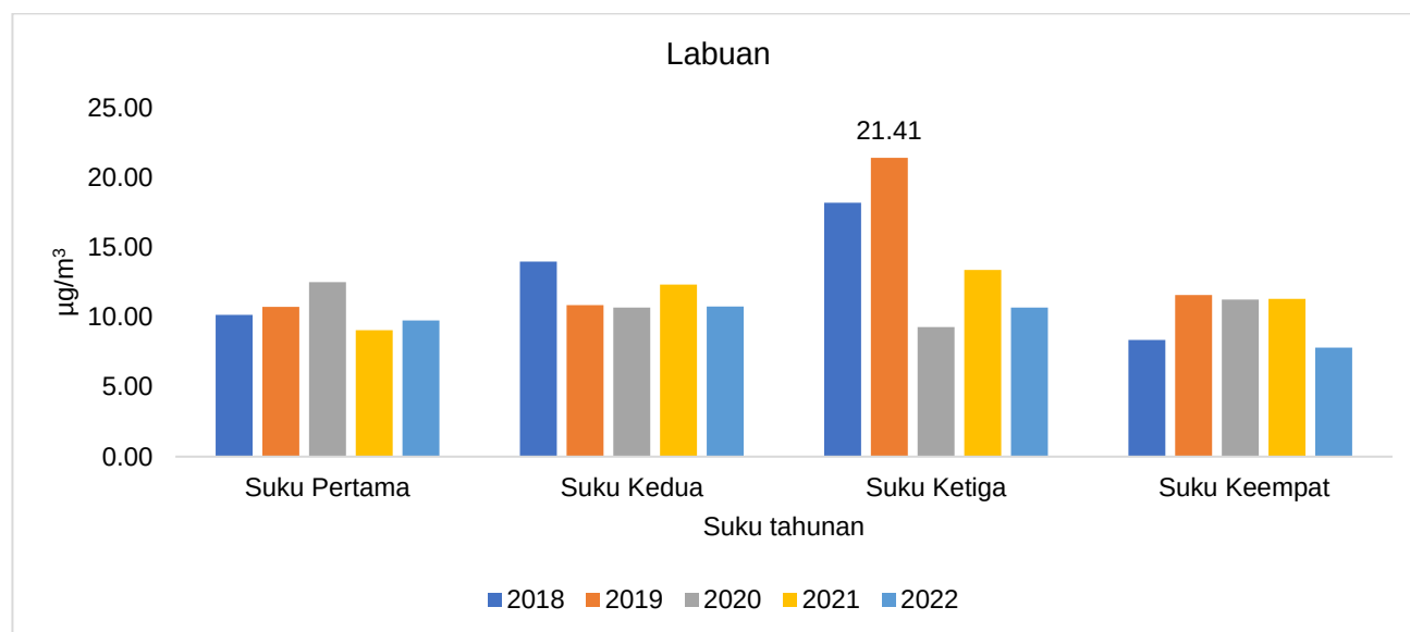
Carta 1.3: Purata suku tahunan kepekatan Habuk Halus ( PM_{2.5} ) dalam udara di stesen Labuan, 2018-2022
