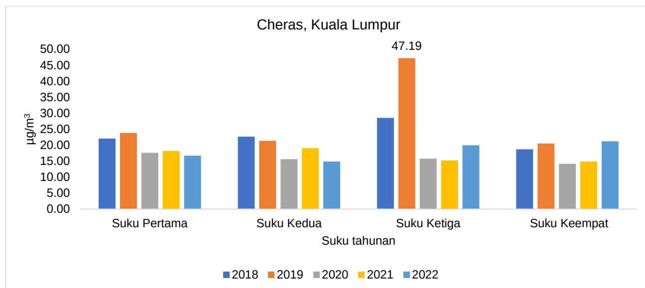
Carta 1.2: Purata suku tahunan kepekatan Habuk Halus ( PM_{2.5} ) dalam udara di stesen Cheras, Kuala Lumpur, 2018-2022
