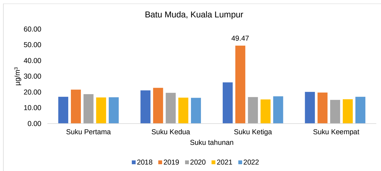
Carta 1.1: Purata suku tahunan kepekatan Habuk Halus ( PM_{2.5} ) dalam udara di stesen Batu Muda, Kuala Lumpur, 2018-2022
