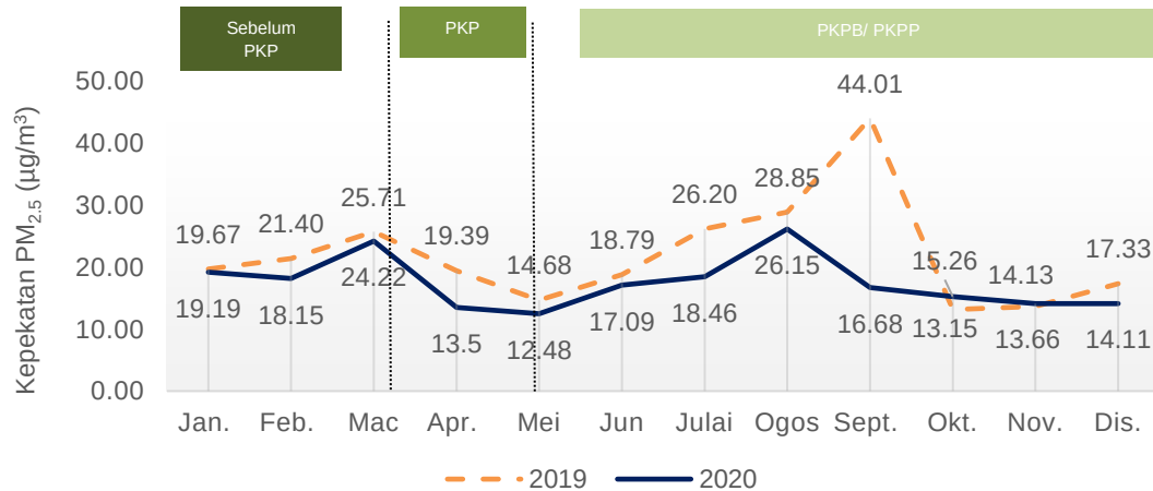
Carta 1.7: Purata bulanan kepekatan PM 2.5 di udara, stesen Seberang Jaya, Pulau Pinang, 2019 dan 2020
