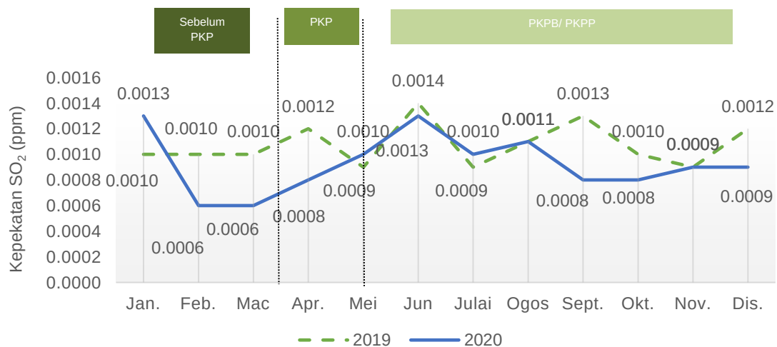
Carta 1.17: Purata bulanan kepekatan SO 2 di udara, stesen Balik Pulau, Pulau Pinang, 2019 dan 2020
