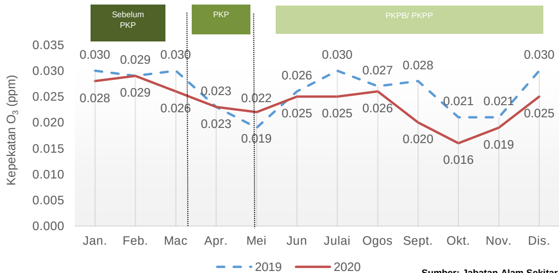
Carta 1.9: Purata bulanan kepekatan O 3 di udara, stesen Balik Pulau, Pulau Pinang, 2019 dan 2020
