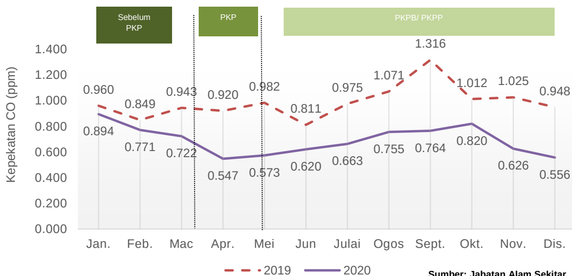
Carta 1.15: Purata bulanan kepekatan CO di udara, stesen Seberang Jaya, Pulau Pinang, 2019 dan 2020
