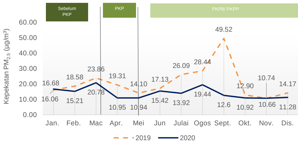
Carta 1.8: Purata bulanan kepekatan PM 2.5 di udara, stesen USM, Pulau Pinang, 2019 dan 2020
