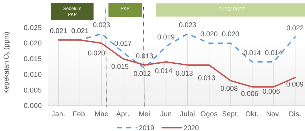
Carta 1.10: Purata bulanan kepekatan O 3 di udara, stesen Perai, Pulau Pinang, 2019 dan 2020
