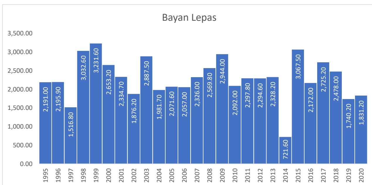
Carta1.1: Taburan hujan di stesen meteorologi Bayan Lepas, Pulau Pinang, 1995-2020
