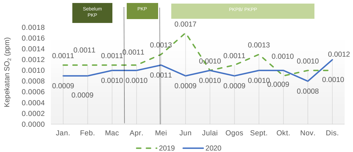
Carta 1.19: Purata bulanan kepekatan SO 2 di udara, stesen Seberang Jaya, Pulau Pinang, 2019 dan 2020
