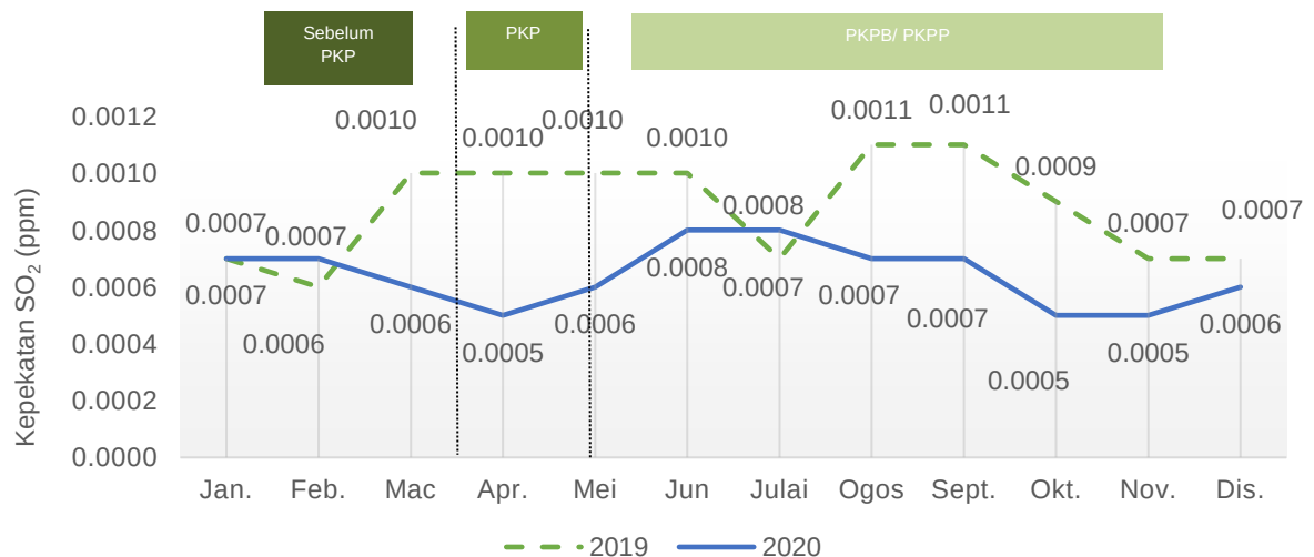
Carta 1.18: Purata bulanan kepekatan SO 2 di udara, stesen Perai, Pulau Pinang, 2019 dan 2020
