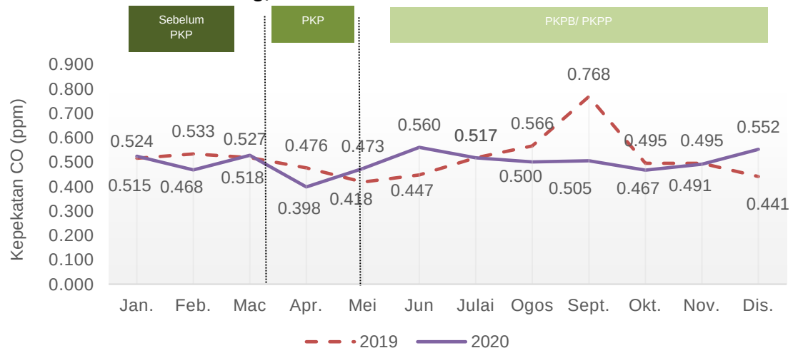
Carta 1.13: Purata bulanan kepekatan CO di udara, stesen Balik Pulau, Pulau Pinang, 2019 dan 2020
