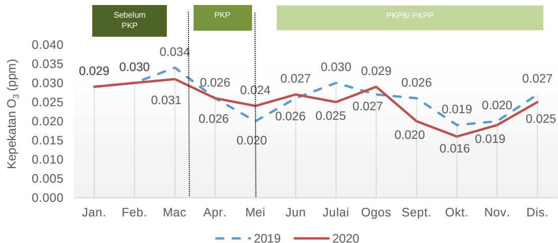
Carta 1.12: Purata bulanan kepekatan O 3 di udara, stesen USM, Pulau Pinang, 2019 dan 2020
