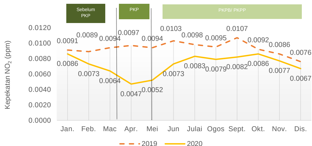
Carta 1.23: Purata bulanan kepekatan NO 2 di udara, stesen Seberang Jaya, Pulau Pinang, 2019 dan 2020
