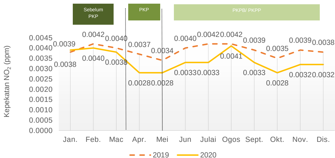
Carta 1.21: Purata bulanan kepekatan NO 2 di udara, stesen Balik Pulau, Pulau Pinang, 2019 dan 2020
