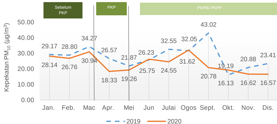
Carta 1.2: Purata bulanan kepekatan PM 10 di udara, stesen Perai, Pulau Pinang, 2019 dan 2020
