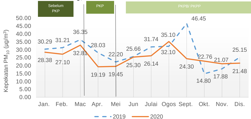
Carta 1.3: Purata bulanan kepekatan PM 10 di udara, stesen Seberang Jaya, Pulau Pinang, 2019 dan 2020
