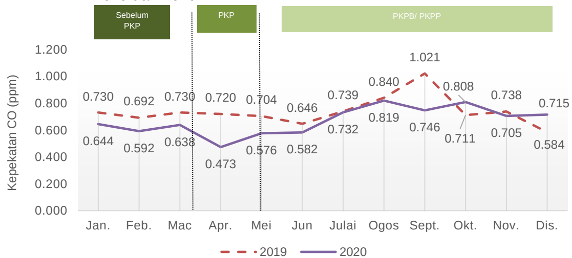
Carta 1.14: Purata bulanan kepekatan CO di udara, stesen Perai, Pulau Pinang, 2019 dan 2020
