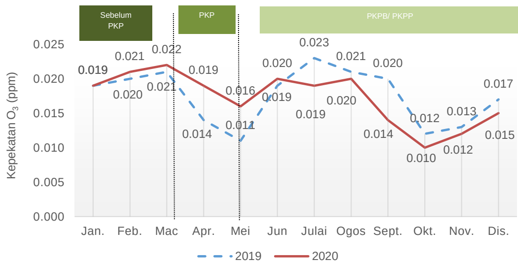
Carta 1.11: Purata bulanan kepekatan O 3 di udara, stesen Seberang Jaya, Pulau Pinang, 2019 dan 2020
