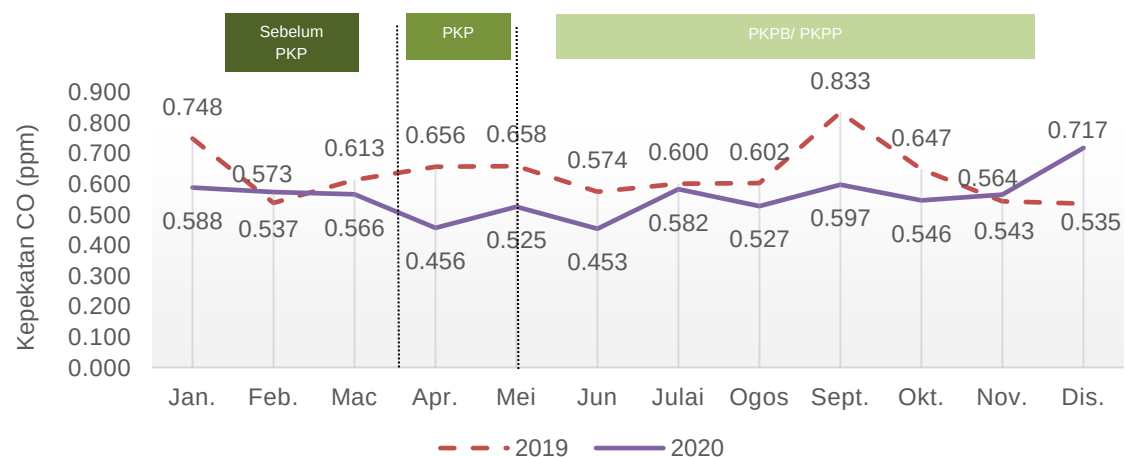
Carta 1.16: Purata bulanan kepekatan CO di udara, stesen USM, Pulau Pinang, 2019 dan 2020
