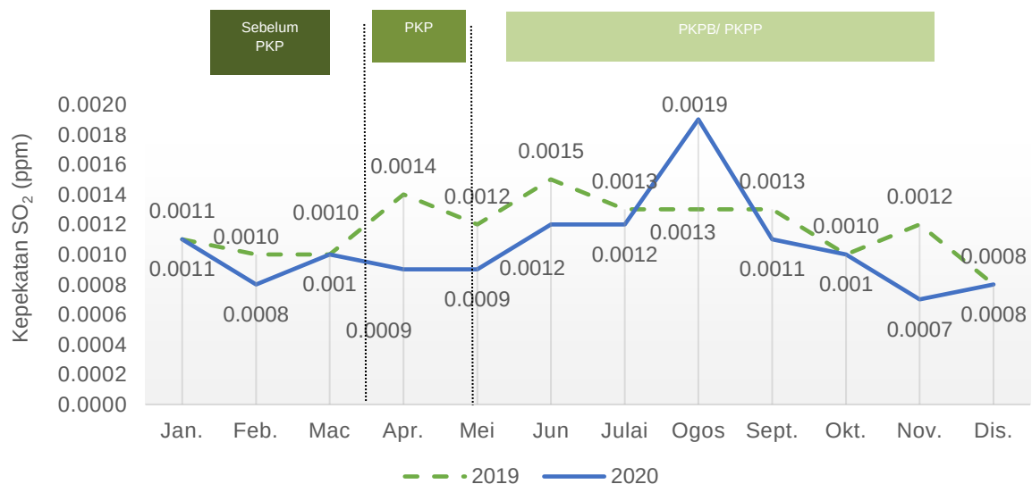
Carta 1.20: Purata bulanan kepekatan SO 2 di udara, stesen USM, Pulau Pinang, 2019 dan 2020
