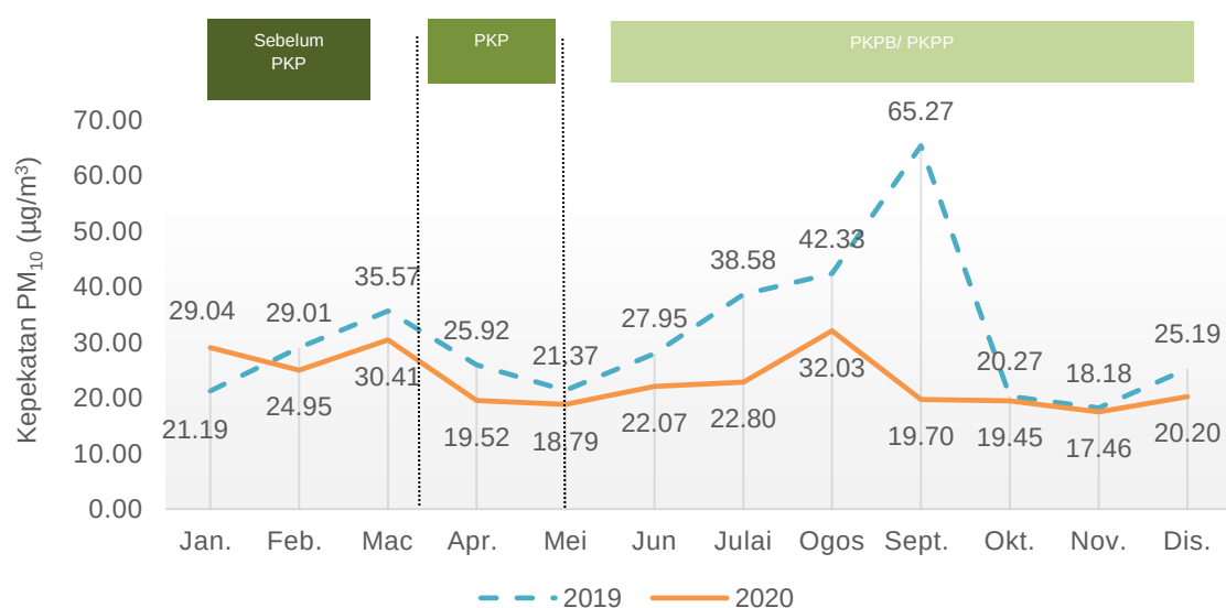
Carta 1.1: Purata bulanan kepekatan PM_{10} di udara, stesen Balik Pulau, Pulau Pinang, 2019 dan 2020
