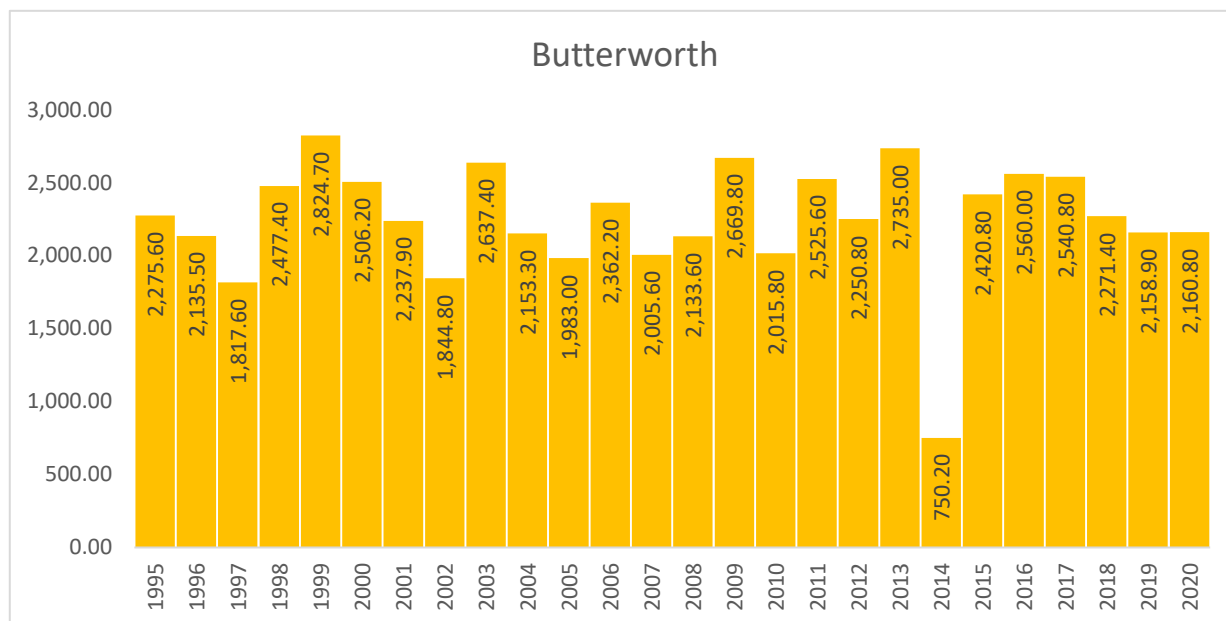
Carta 1.2: Taburan hujan di stesen meteorologi Butterworth, Pulau Pinang, 1995 - 2020
