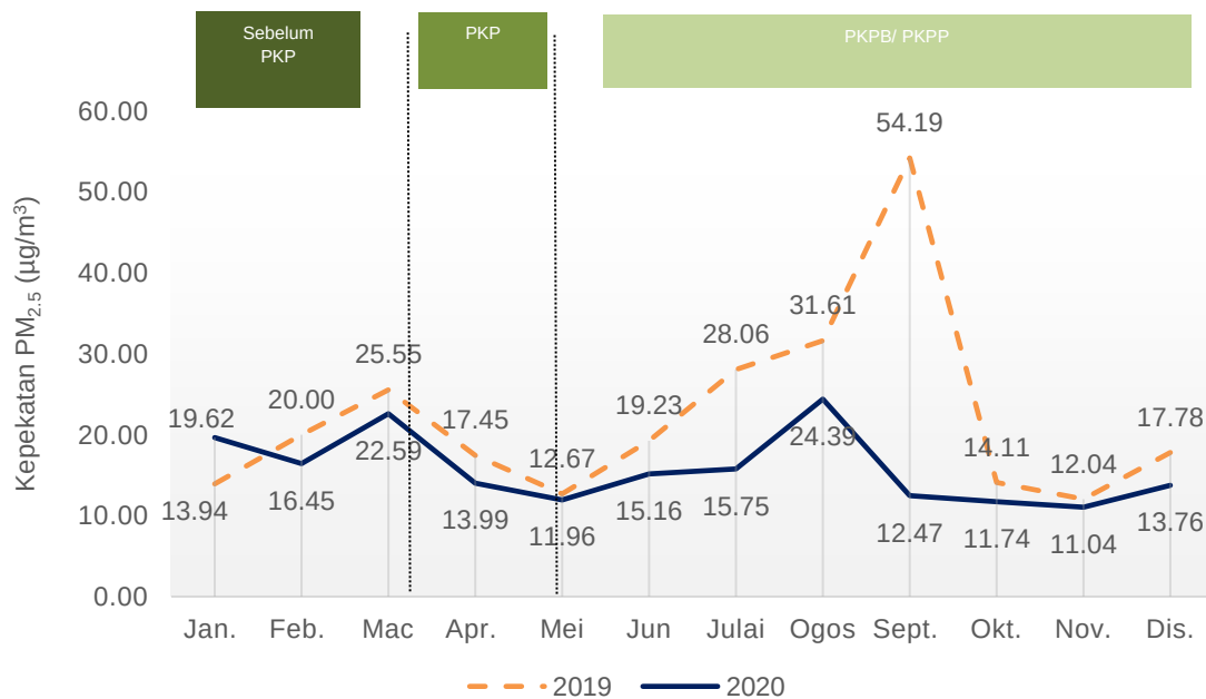
Carta 1.5: Purata bulanan kepekatan PM_{2.5} di udara, stesen Balik Pulau, Pulau Pinang, 2019 dan 2020
