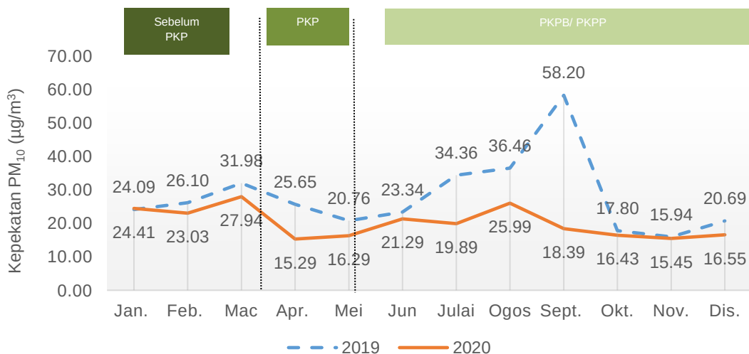
Carta 1.4: Purata bulanan kepekatan PM 10 di udara, stesen USM, Pulau Pinang, 2019 dan 2020
