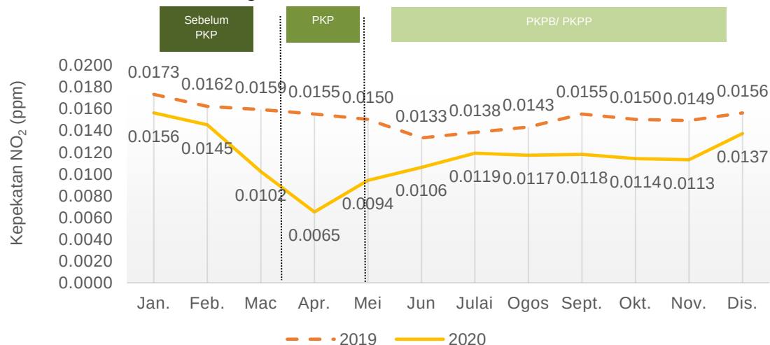
Carta 1.23: Purata bulanan kepekatan NO 2 di udara, stesen Seberang Jaya, Pulau Pinang, 2019 dan 2020
