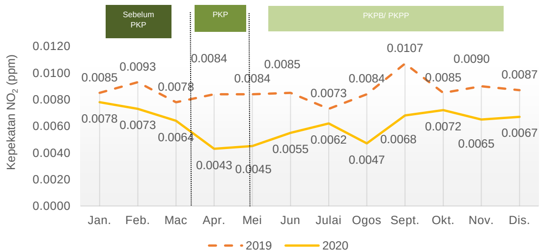
Carta 1.24: Purata bulanan kepekatan NO 2 di udara, stesen USM, Pulau Pinang, 2019 dan 2020
