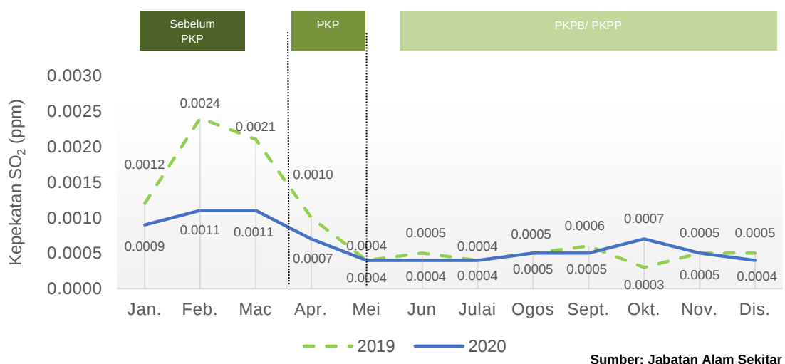
Carta 1.36: Purata bulanan kepekatan SO 2 di udara, stesen Samalaju, Sarawak, 2019 dan 2020
