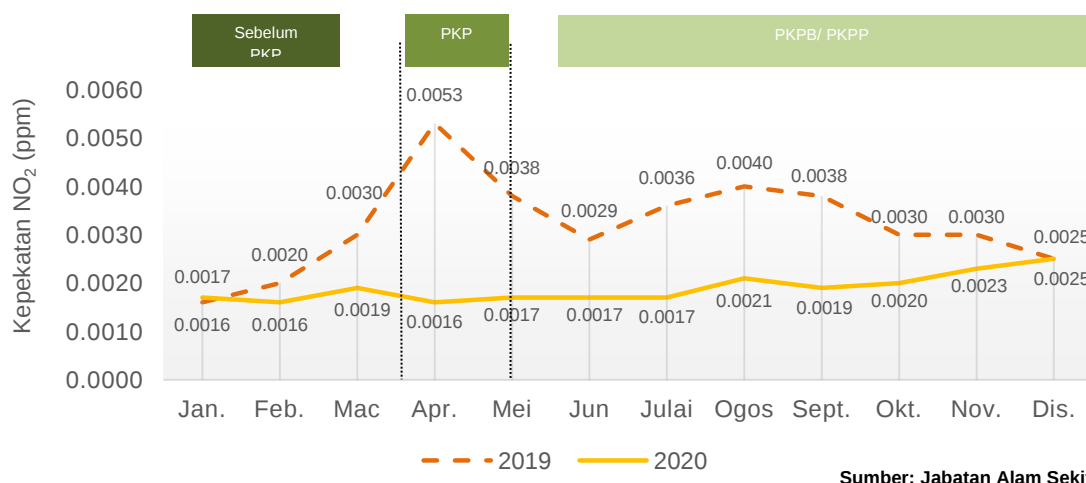
Carta 1.41: Purata bulanan kepekatan NO 2 di udara, stesen Samalaju, Sarawak, 2019 dan 2020
