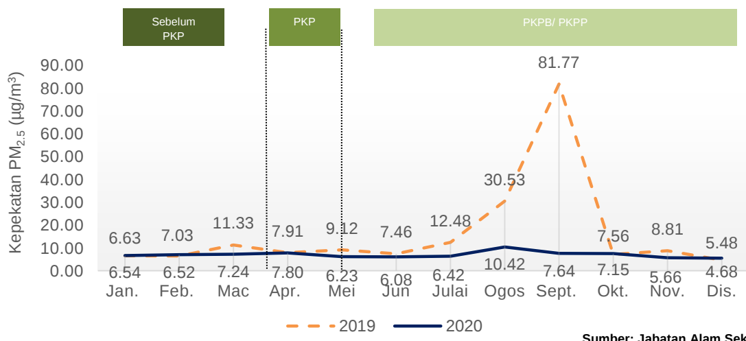
Carta 1.21: Purata bulanan kepekatan PM 2.5 di udara, stesen Samarahan, Sarawak, 2019 dan 2020
