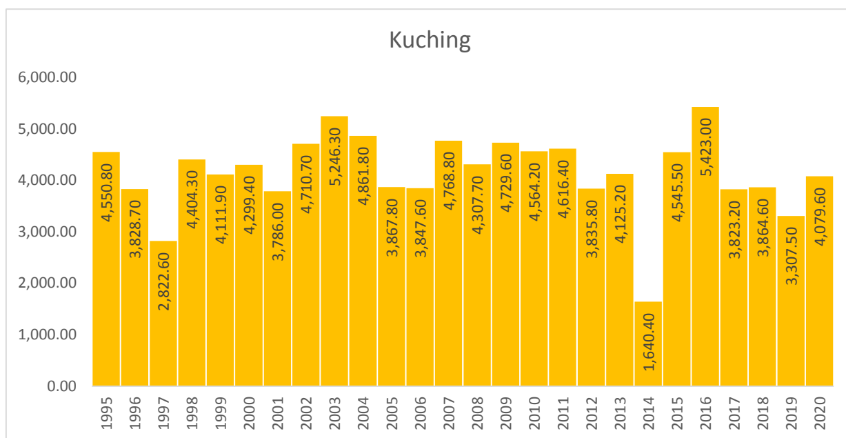
Carta 1.2: Taburan hujan di stesen meteorologi Kuching, Sarawak, 1995 - 2020
