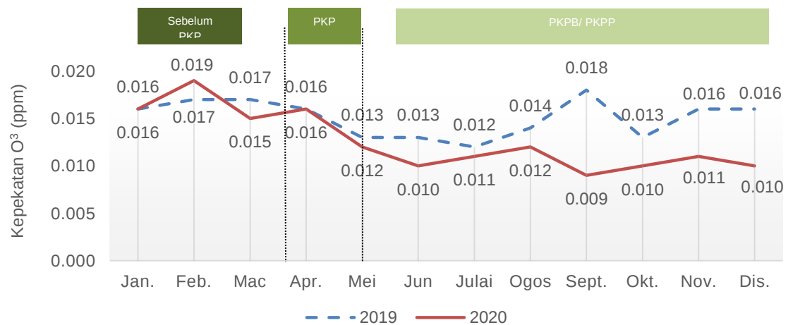
Carta 1.25: Purata bulanan kepekatan O 3 di udara, stesen Bintulu, Sarawak, 2019 dan 2020
