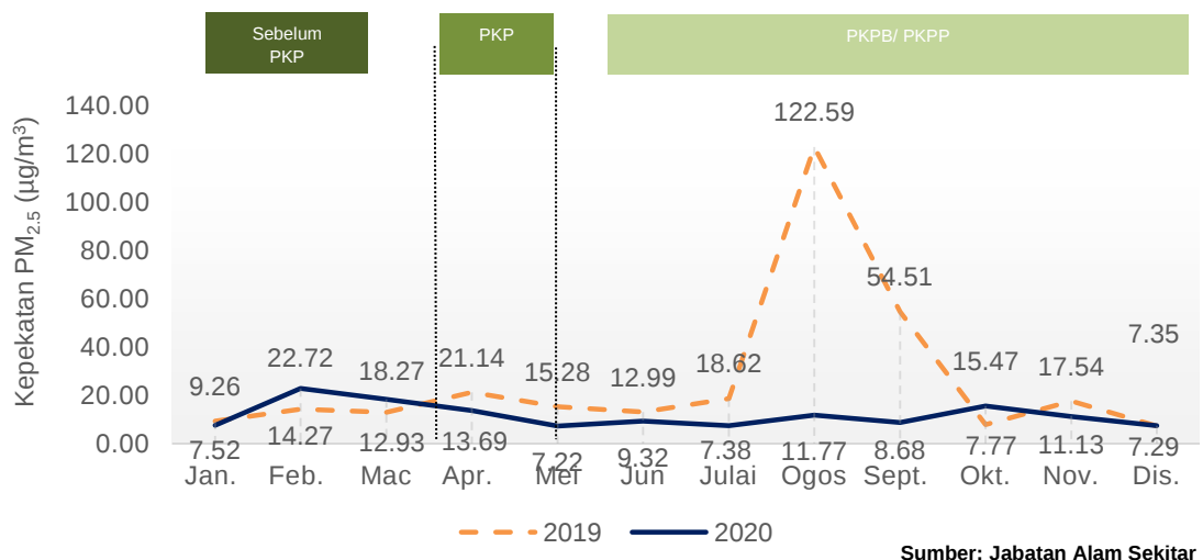
Carta 1.14: Purata bulanan kepekatan PM 2.5 di udara, stesen ILP Miri, Sarawak, 2019 dan 2020
