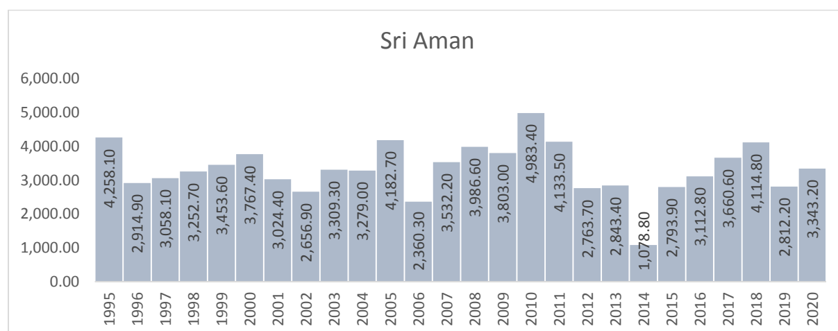
Carta 1.5: Taburan hujan di stesen meteorologi Sri Aman, Sarawak, 1995 – 2020
