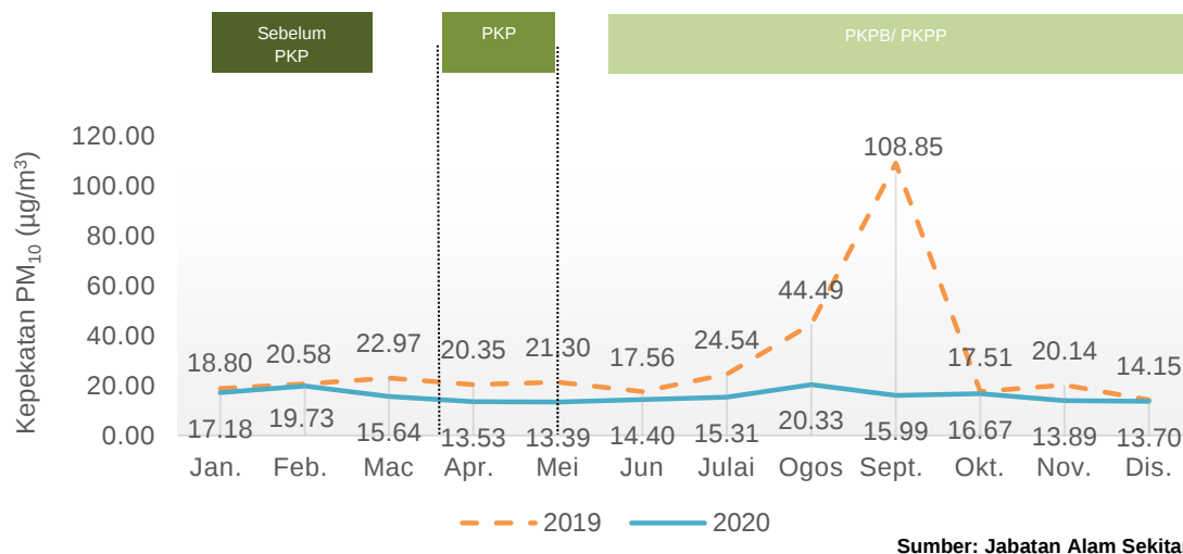
Carta 1.4: Purata bulanan kepekatan PM 10 di udara, stesen Kuching, Sarawak, 2019 dan 2020
