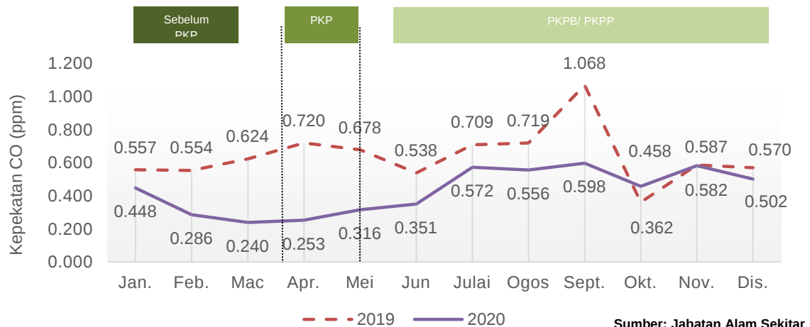
Carta 1.32: Purata bulanan kepekatan CO di udara, stesen Sibu, Sarawak, 2019 dan 2020
