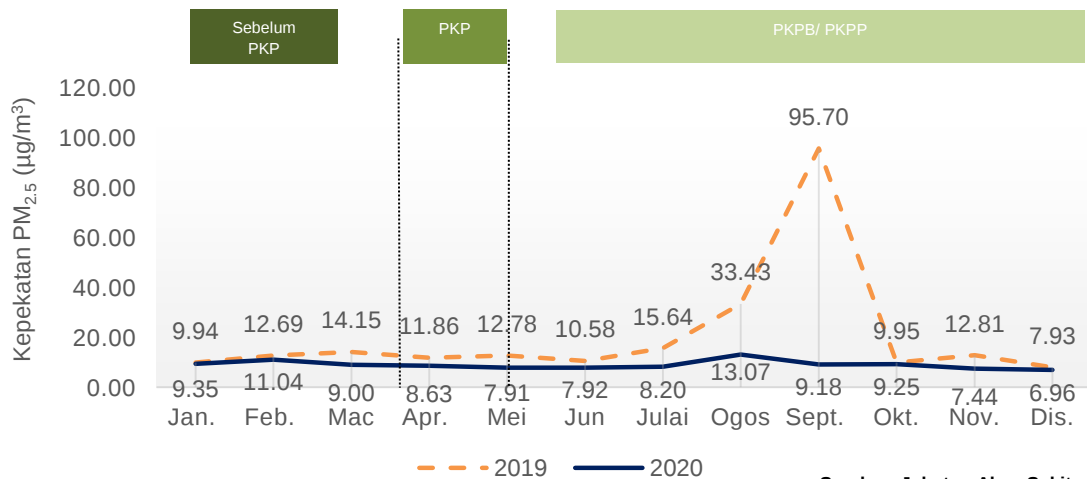
Carta 1.16: Purata bulanan kepekatan PM_{2.5} di udara, stesen Kuching, Sarawak, 2019 dan 2020
