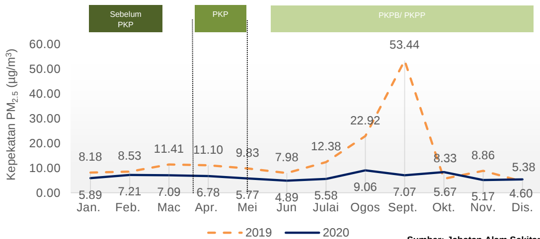
Carta 1.19: Purata bulanan kepekatan PM 2.5 di udara, stesen Mukah, Sarawak, 2019 dan 2020
