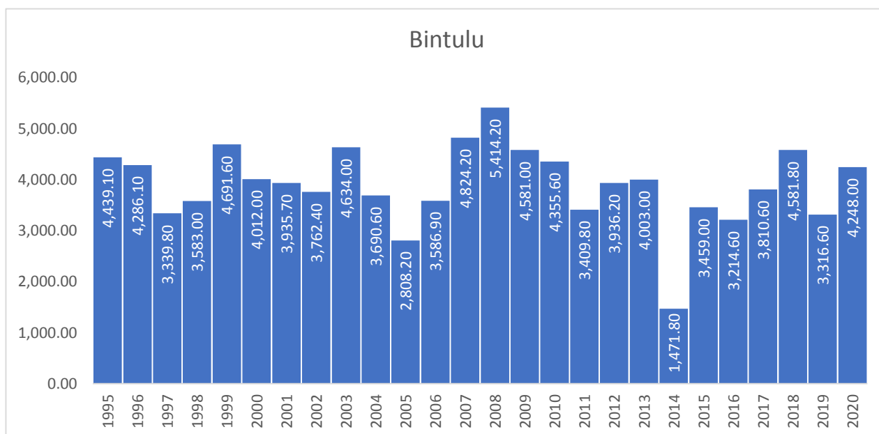
Carta 1.1: Taburan hujan di stesen meteorologi Bintulu, Sarawak, 1995-2020
