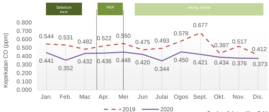
Carta 1.29: Purata bulanan kepekatan CO di udara, stesen Bintulu, Sarawak, 2019 dan 2020
