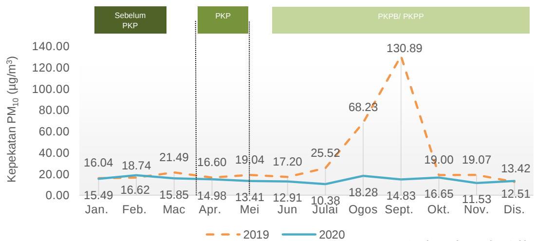
Carta 1.12: Purata bulanan kepekatan PM 10 di udara, stesen Sri Aman, Sarawak, 2019 dan 2020
