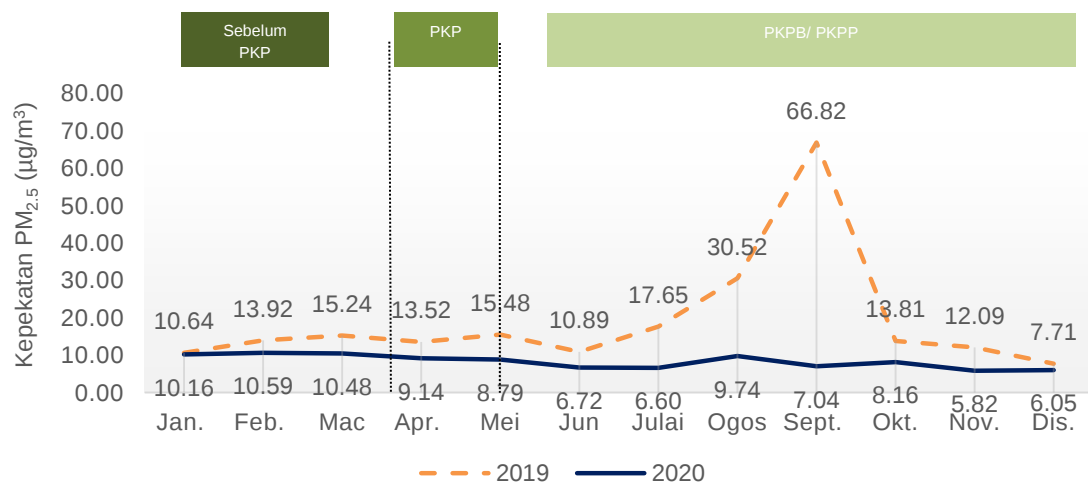
Carta 1.23: Purata bulanan kepekatan PM 2.5 di udara, stesen Sibu, Sarawak, 2019 dan 2020
