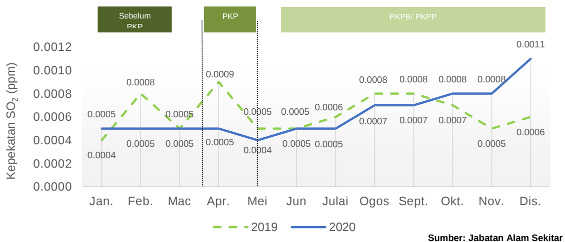
Carta 1.35: Purata bulanan kepekatan SO 2 di udara, stesen Miri, Sarawak, 2019 dan 2020
