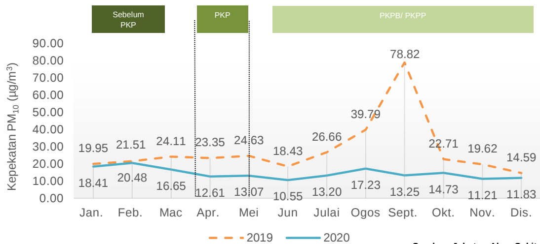
Carta 1.11: Purata bulanan kepekatan PM 10 di udara, stesen Sibul, Sarawak, 2019 dan 2020
