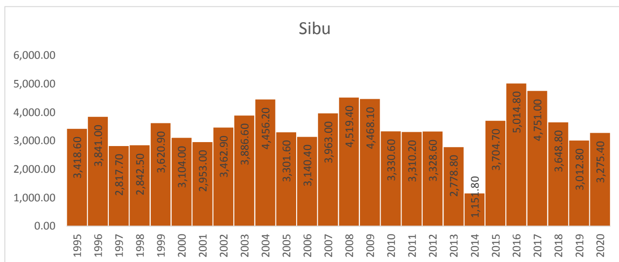
Carta 1.4: Taburan hujan di stesen meteorologi Sibul, Sarawak, 1995 – 2020
