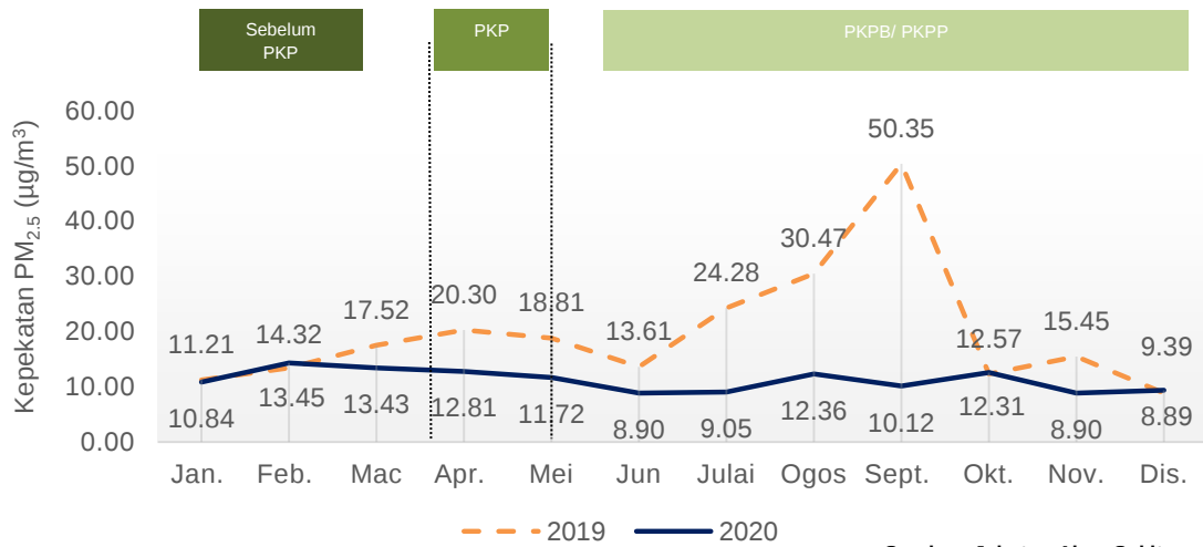
Carta 1.13: Purata bulanan kepekatan PM 2.5 di udara, stesen Bintulu, Sarawak, 2019 dan 2020
