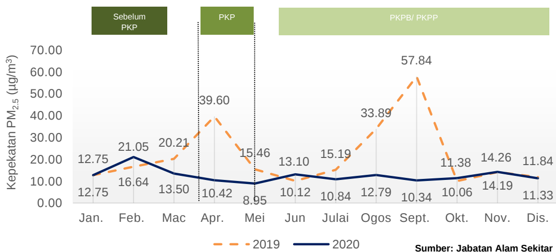
Carta 1.18: Purata bulanan kepekatan PM_{2.5} di udara, stesen Miri, Sarawak, 2019 dan 2020
