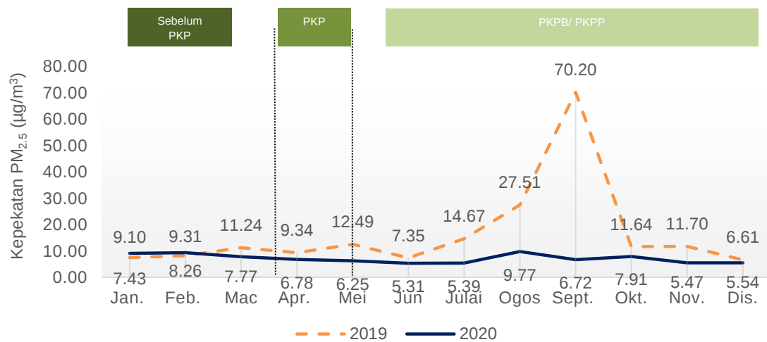
Carta 1.22: Purata bulanan kepekatan PM 2.5 di udara, stesen Sarikei, Sarawak, 2019 dan 2020
