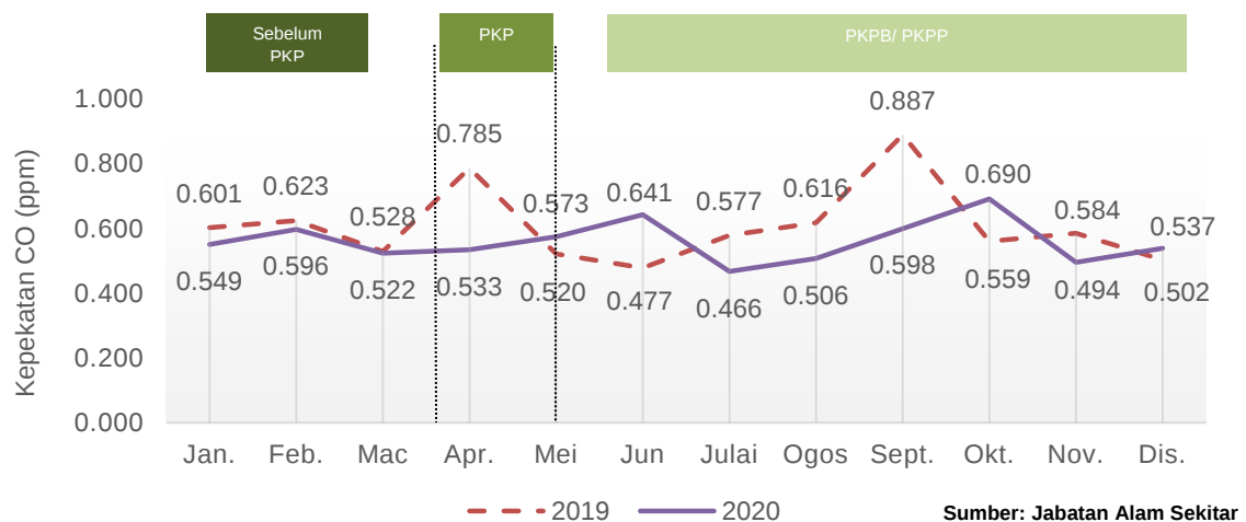
Carta 1.31: Purata bulanan kepekatan CO di udara, stesen Miri, Sarawak, 2019 dan 2020
