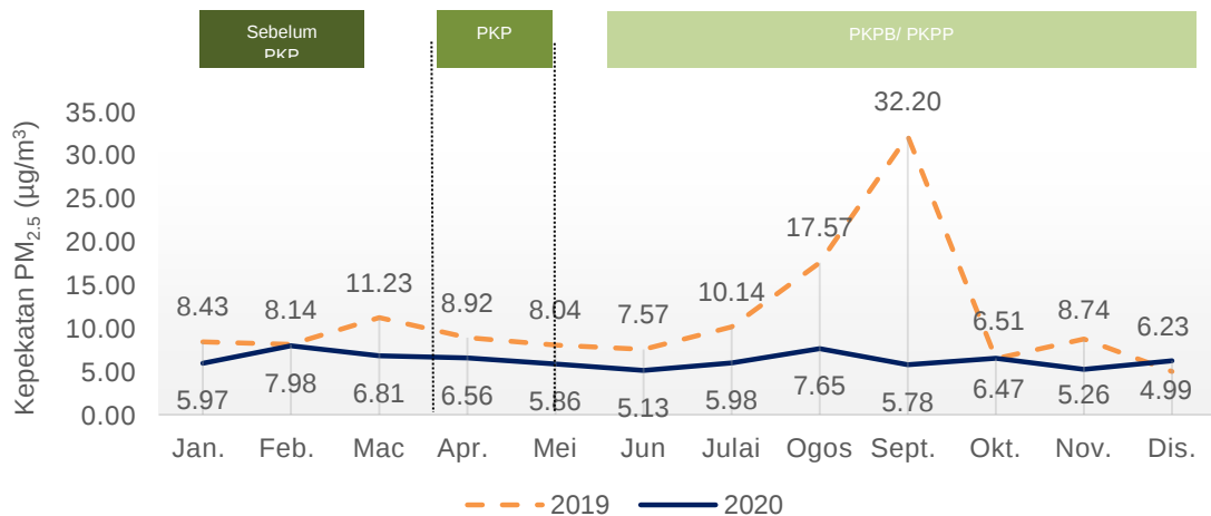
Carta 1.15: Purata bulanan kepekatan PM 2.5 di udara, stesen Kapit, Sarawak, 2019 dan 2020
