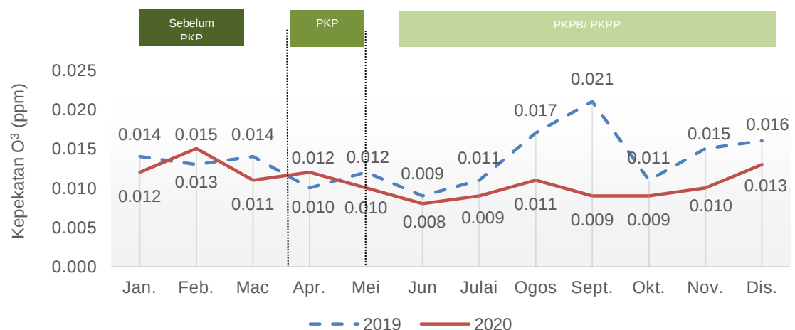
Carta 1.26: Purata bulanan kepekatan O 3 di udara, stesen Kuching, Sarawak, 2019 dan 2020
