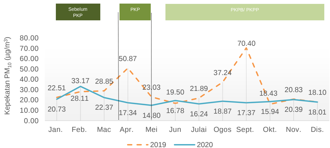
Carta 1.6: Purata bulanan kepekatan PM 10 di udara, stesen Miri, Sarawak, 2019 dan 2020
