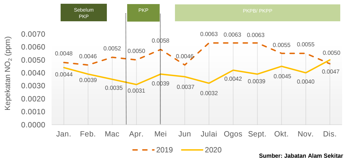
Carta 1.38: Purata bulanan kepekatan NO 2 di udara, stesen Bintulu, Sarawak, 2019 dan 2020
