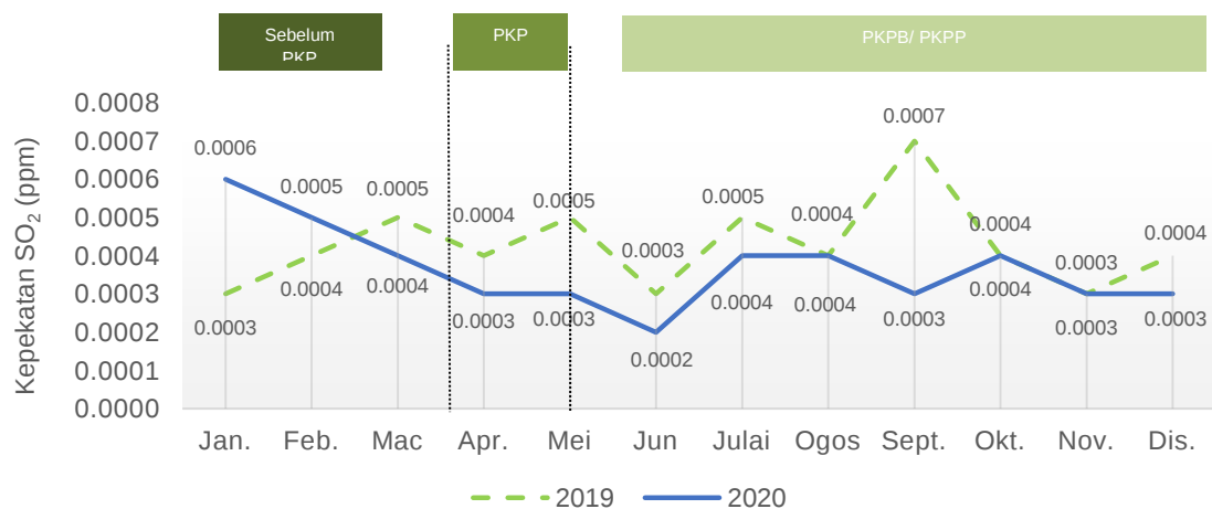
Carta 1.33: Purata bulanan kepekatan SO 2 di udara, stesen Bintulu, Sarawak, 2019 dan 2020
