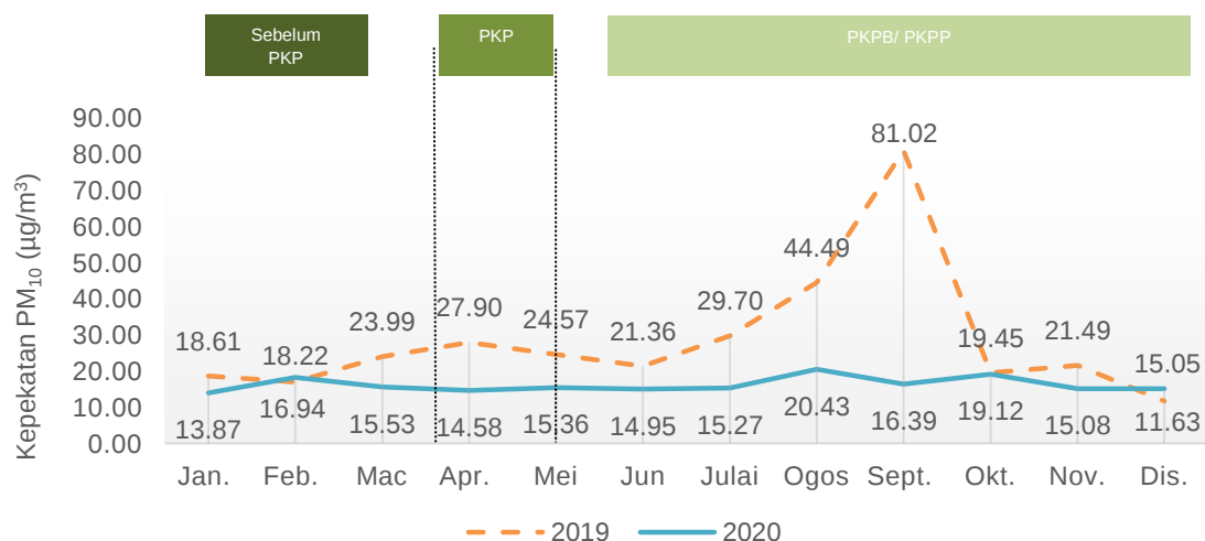
Carta 1.7: Purata bulanan kepekatan PM 10 di udara, stesen Mukah, Sarawak, 2019 dan 2020
