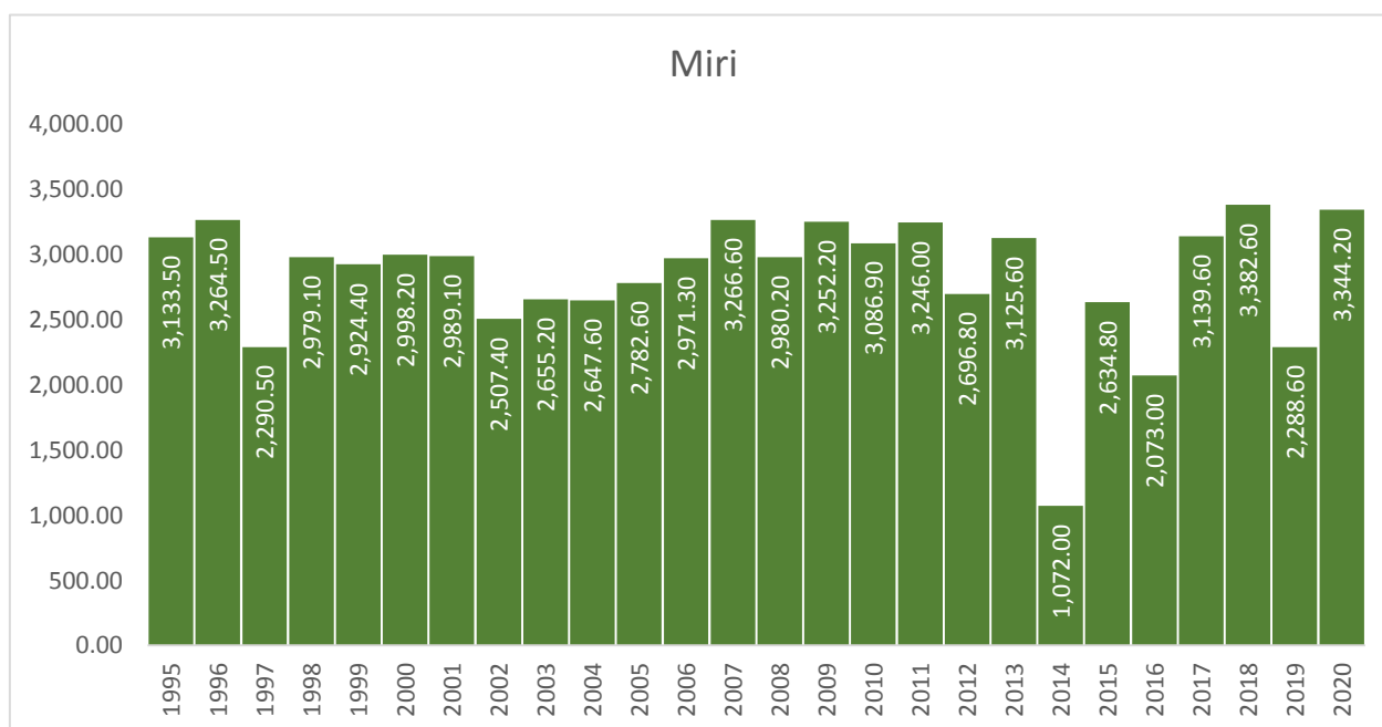
Carta 1.3: Taburan hujan di stesen meteorologi Miri, Sarawak, 1995 – 2020
