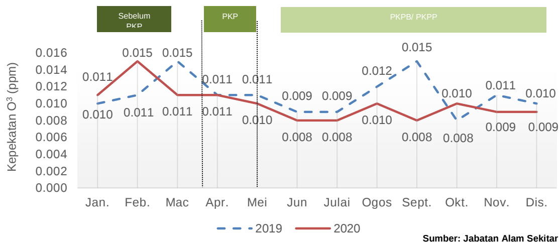
Carta 1.28: Purata bulanan kepekatan O 3 di udara, stesen Sibul, Sarawak, 2019 dan 2020
