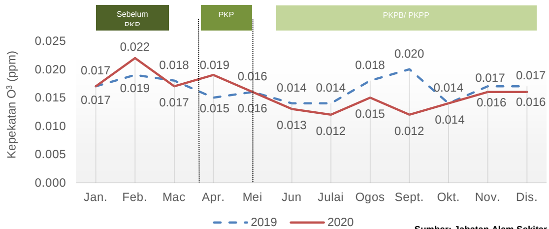
Carta 1.27: Purata bulanan kepekatan O 3 di udara, stesen Miri, Sarawak, 2019 dan 2020
