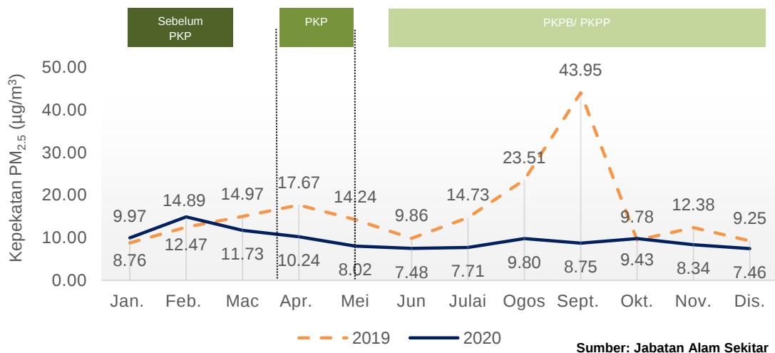
Carta 1.20: Purata bulanan kepekatan PM 2.5 di udara, stesen Samalaju, Sarawak, 2019 dan 2020
