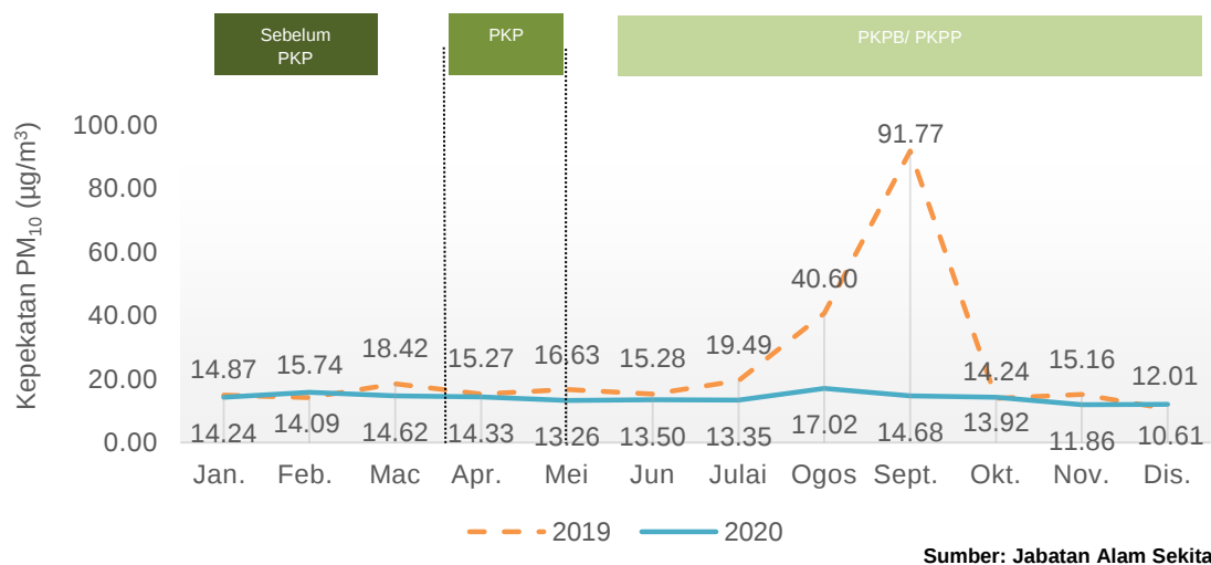
Carta 1.9: Purata bulanan kepekatan PM 10 di udara, stesen Samarahan, Sarawak, 2019 dan 2020
