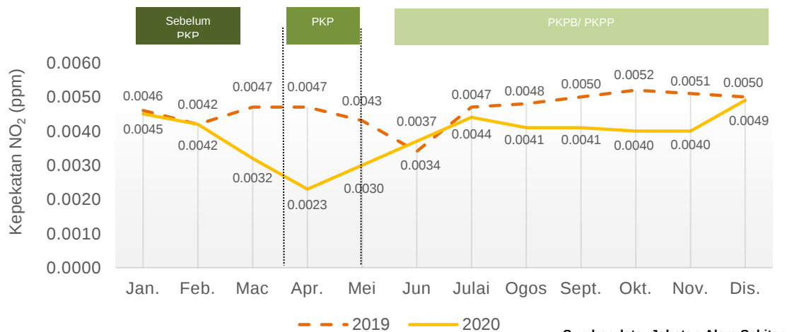
Carta 1.42: Purata bulanan kepekatan NO 2 di udara, stesen Sibul, Sarawak, 2019 dan 2020
