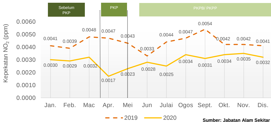
Carta 1.40: Purata bulanan kepekatan NO 2 di udara, stesen Miri, Sarawak, 2019 dan 2020
