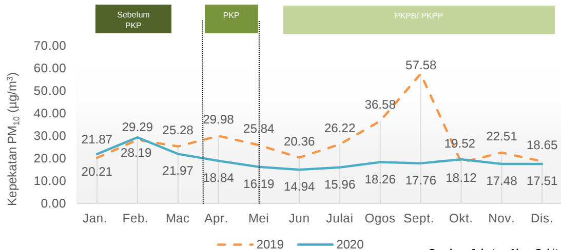
Carta 1.8: Purata bulanan kepekatan PM 10 di udara, stesen Samalaju, Sarawak, 2019 dan 2020
