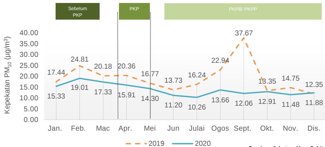
Carta 1.5: Purata bulanan kepekatan PM 10 di udara, stesen Limbang, Sarawak, 2019 dan 2020
