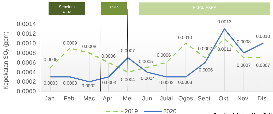
Carta 1.34: Purata bulanan kepekatan SO 2 di udara, stesen Kuching, Sarawak, 2019 dan 2020
