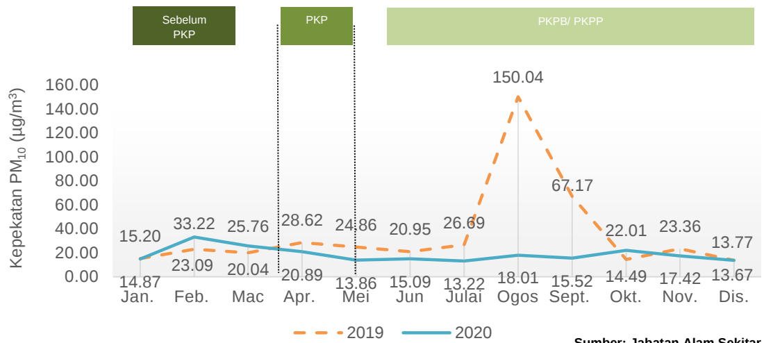
Carta 1.2: Purata bulanan kepekatan PM 10 di udara, stesen ILP Miri, Sarawak, 2019 dan 2020
