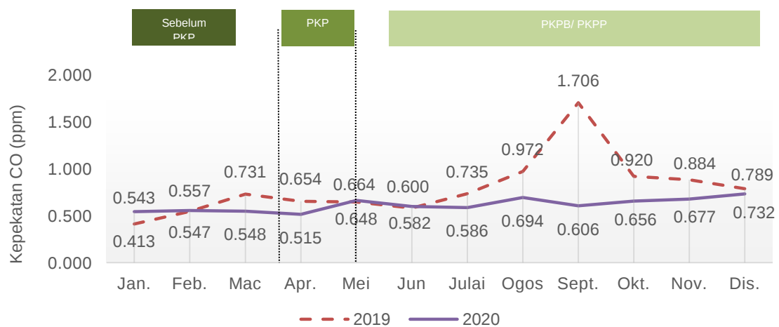
Carta 1.30: Purata bulanan kepekatan CO di udara, stesen Kuching, Sarawak, 2019 dan 2020
