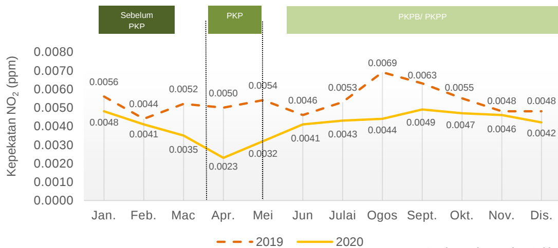
Carta 1.39: Purata bulanan kepekatan NO 2 di udara, stesen Kuching, Sarawak, 2019 dan 2020
