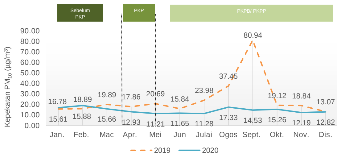
Carta 1.10: Purata bulanan kepekatan PM 10 di udara, stesen Sarikei, Sarawak, 2019 dan 2020
