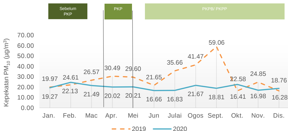
Carta 1.1: Purata bulanan kepekatan PM_{10} di udara, stesen Bintulu, Sarawak, 2019 dan 2020
