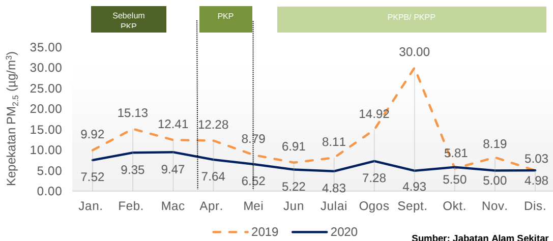
Carta 1.17: Purata bulanan kepekatan PM_{2.5} di udara, stesen Limbang, Sarawak, 2019 dan 2020
