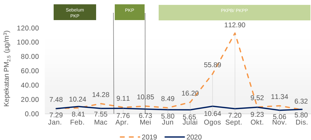
Carta 1.24: Purata bulanan kepekatan PM 2.5 di udara, stesen Sri Aman, Sarawak, 2019 dan 2020
