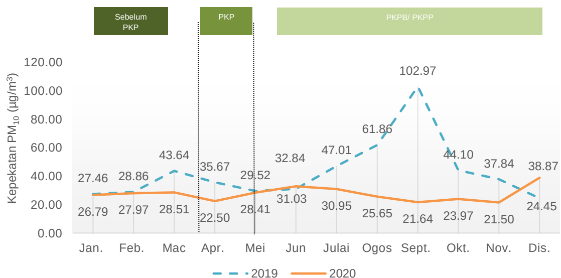
Carta 1.1: Purata bulanan kepekatan PM_{10} di udara, stesen Nilai, Negeri Sembilan, 2019 dan 2020
