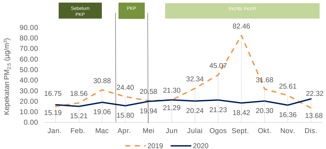
Carta 1.4: Purata bulanan kepekatan PM 2.5 di udara, stesen Nilai, Negeri Sembilan, 2019 dan 2020
