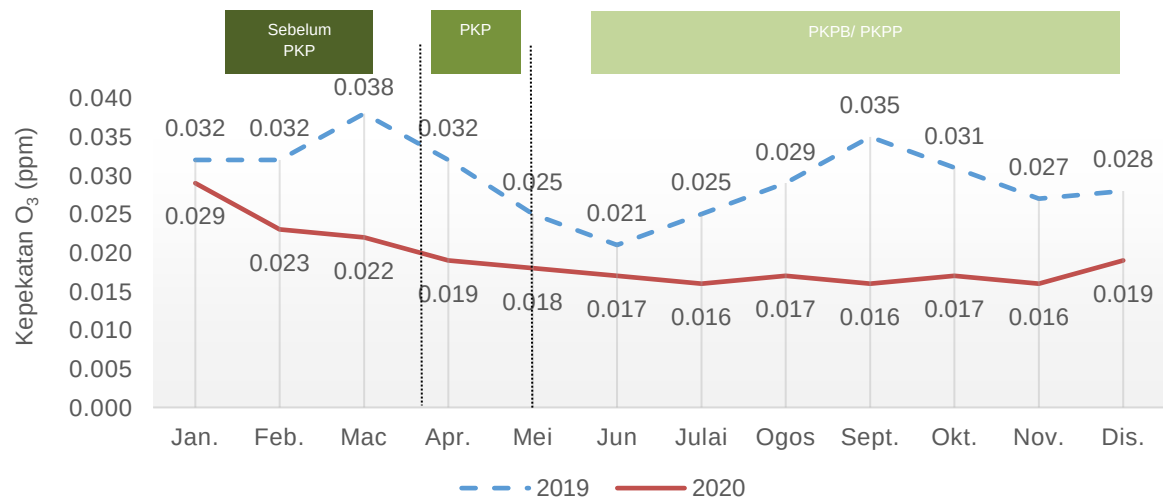
Carta 1.8: Purata bulanan kepekatan O 3 di udara, stesen Port Dickson, Negeri Sembilan, 2019 dan 2020
