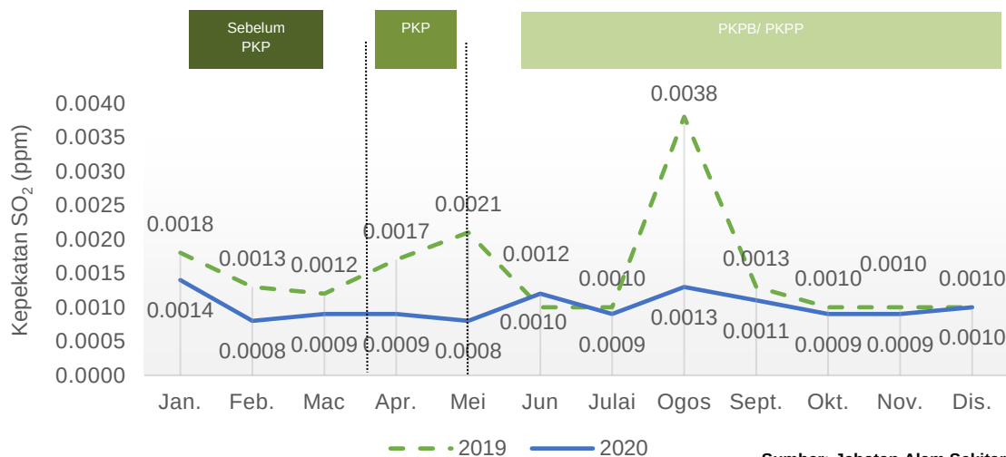
Carta 1.13: Purata bulanan kepekatan SO 2 di udara, stesen Nilai, Negeri Sembilan, 2019 dan 2020
