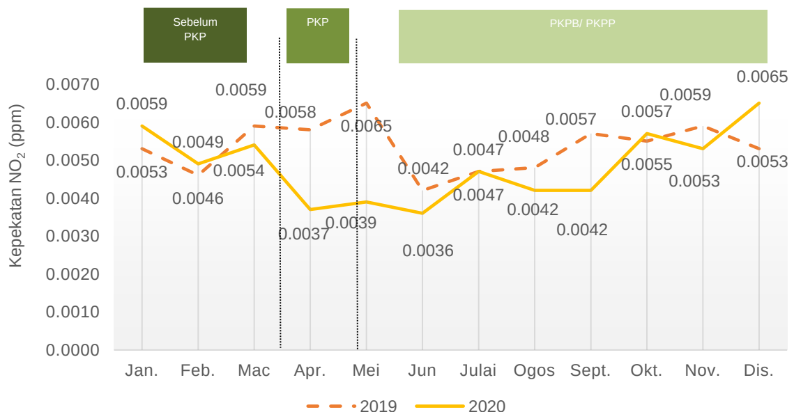
Carta 1.17: Purata bulanan kepekatan NO 2 di udara, stesen Port Dickson, Negeri Sembilan, 2019 dan 2020
