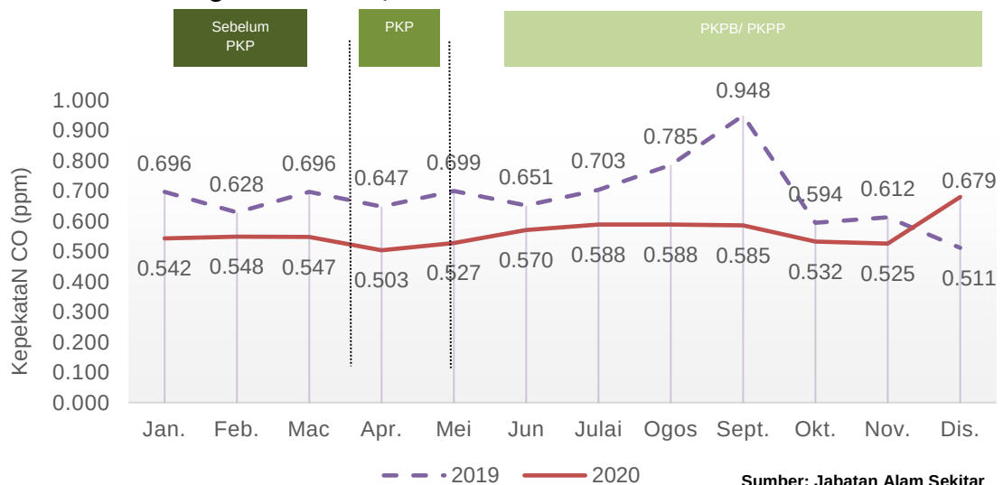
Carta 1.12: Purata bulanan kepekatan CO di udara, stesen Seremban, Negeri Sembilan, 2019 dan 2020
