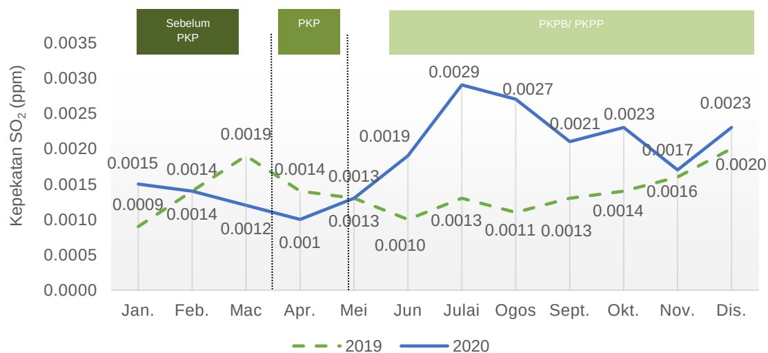
Carta 1.15: Purata bulanan kepekatan SO 2 di udara, stesen Seremban, Negeri Sembilan, 2019 dan 2020
