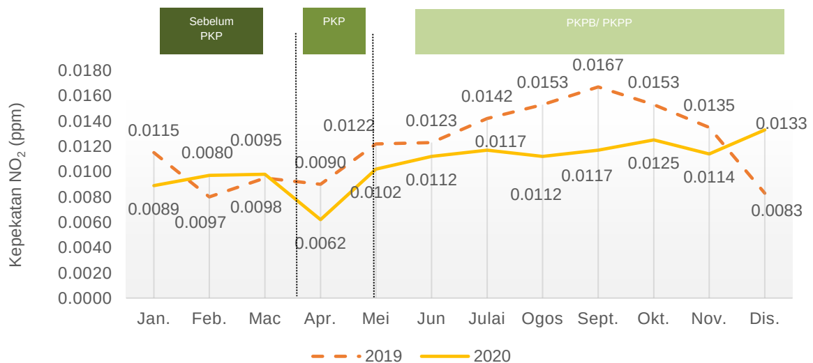
Carta 1.16: Purata bulanan kepekatan NO 2 di udara, stesen Nilai, Negeri Sembilan, 2019 dan 2020
