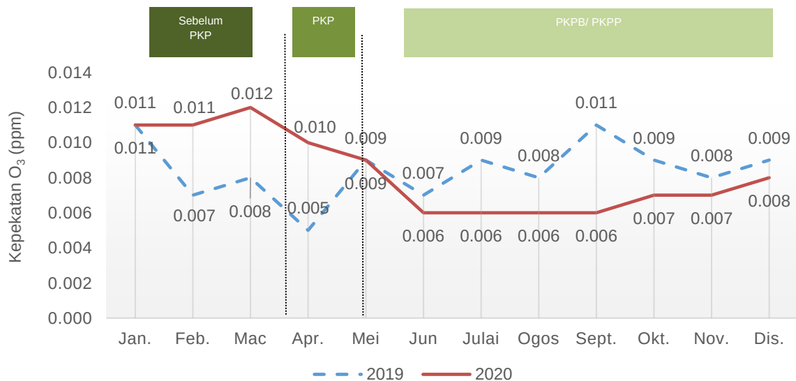
Carta 1.7: Purata bulanan kepekatan O 3 di udara, stesen Nilai, Negeri Sembilan, 2019 dan 2020
