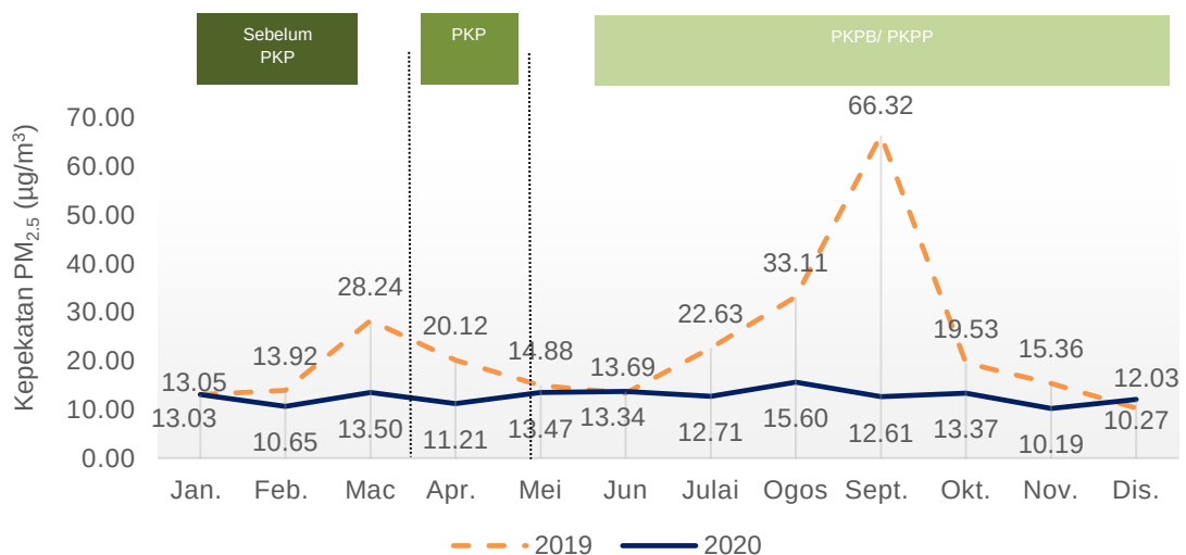
Carta 1.6: Purata bulanan kepekatan PM 2.5 di udara, stesen Seremban, Negeri Sembilan, 2019 dan 2020
