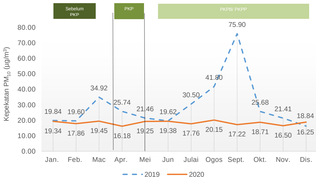
Carta 1.3: Purata bulanan kepekatan PM 10 di udara, stesen Seremban, Negeri Sembilan, 2019 dan 2020
