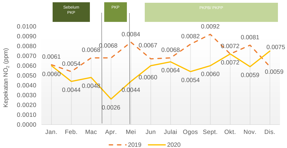
Carta 1.18: Purata bulanan kepekatan NO 2 di udara, stesen Seremban, Negeri Sembilan, 2019 dan 2020
