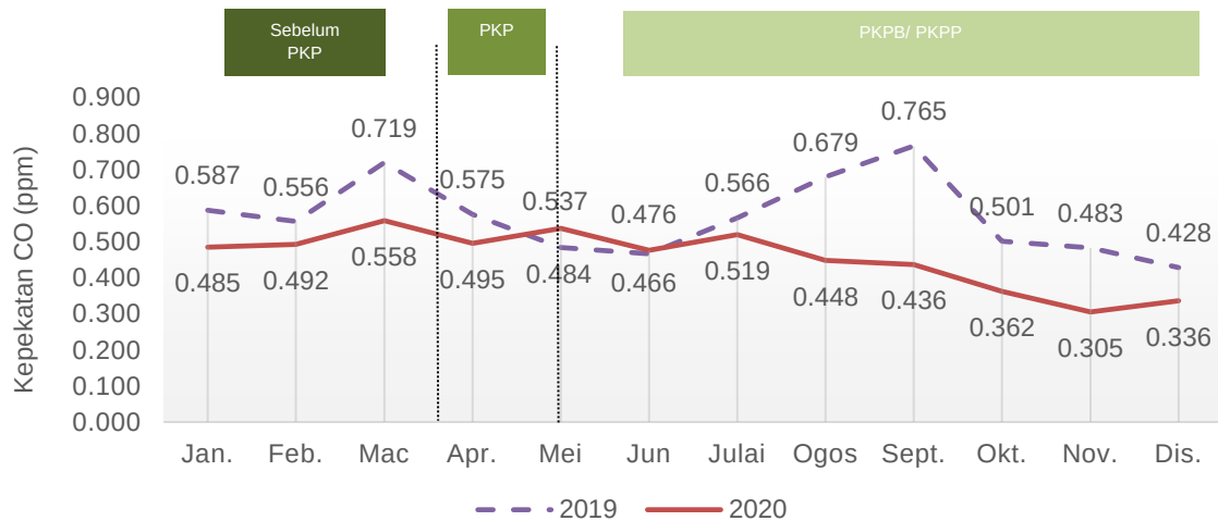
Carta 1.11: Purata bulanan kepekatan CO di udara, stesen Port Dickson, Negeri Sembilan, 2019 dan 2020
