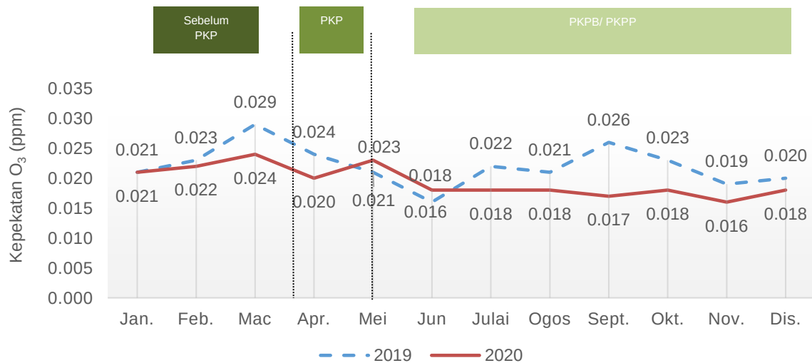
Carta 1.9: Purata bulanan kepekatan O 3 di udara, stesen Seremban, Negeri Sembilan, 2019 dan 2020
