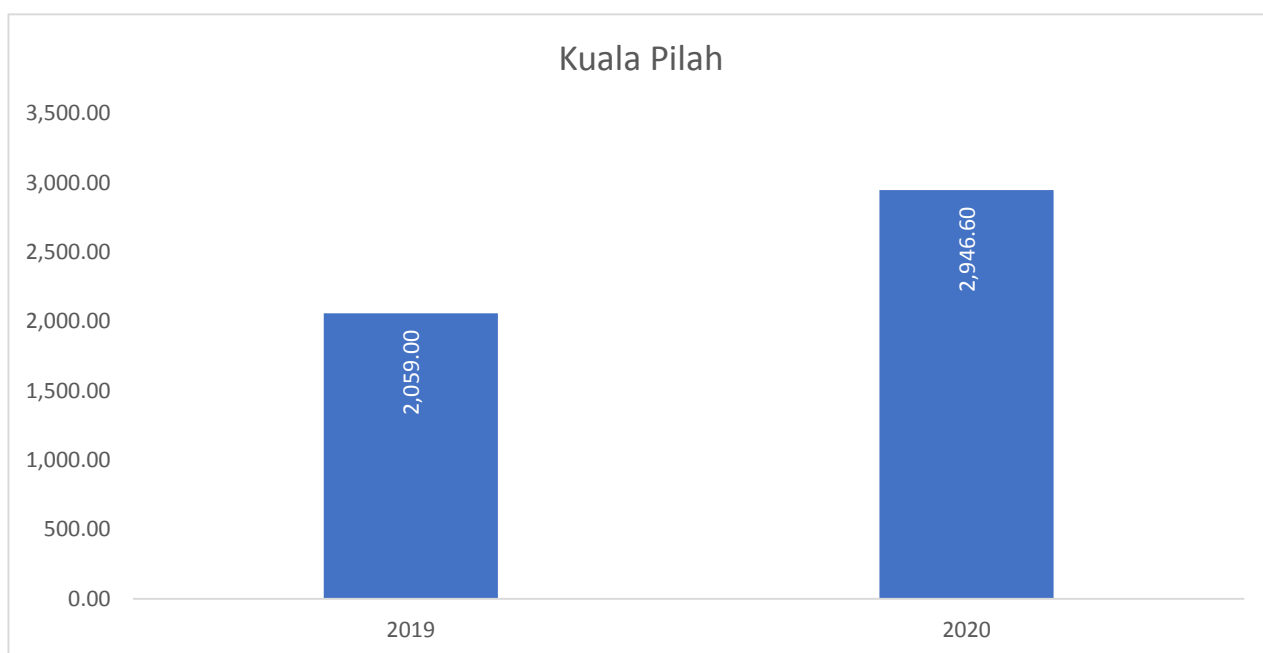
Carta1.1: Taburan hujan di stesen meteorologi Kuala Pilah, Negeri Sembilan, 2019 dan 2020
