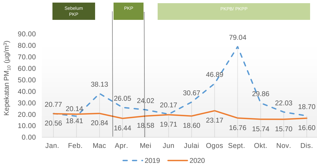
Carta 1.2: Purata bulanan kepekatan PM 10 di udara, stesen Port Dickson, Negeri Sembilan, 2019 dan 2020
