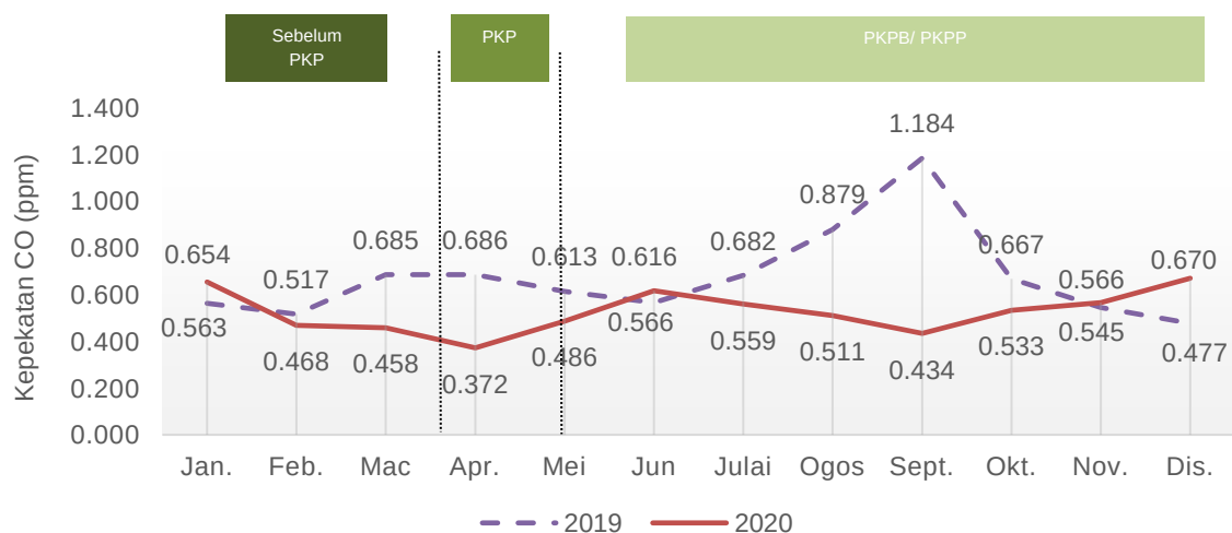
Carta 1.10: Purata bulanan kepekatan CO di udara, stesen Nilai, Negeri Sembilan, 2019 dan 2020
