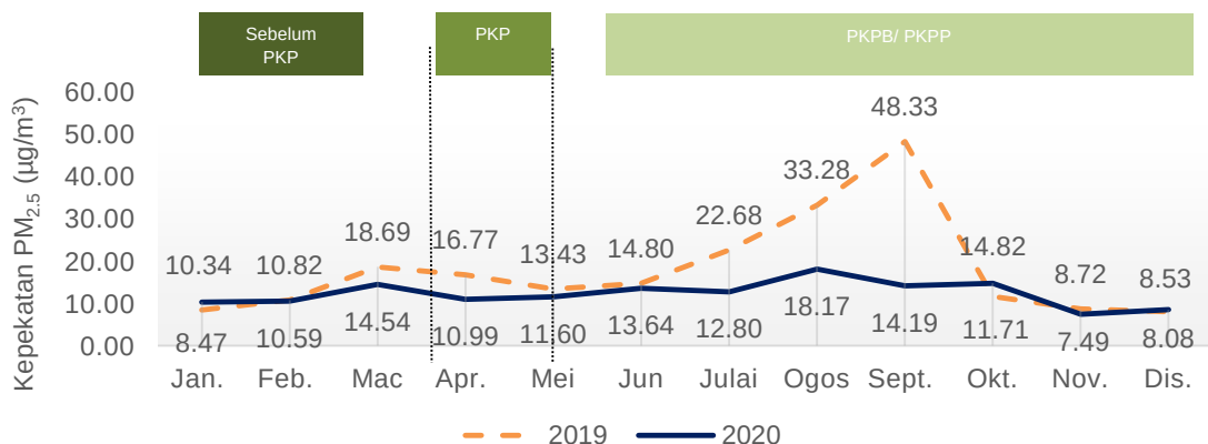
Carta 1.7: Purata bulanan kepekatan PM 2.5 di udara, Stesen Jerantut, Pahang, 2019 dan 2020
