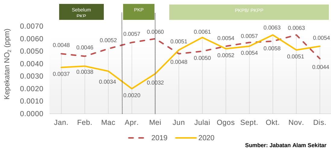
Carta 1.23: Purata bulanan kepekatan NO 2 di udara, stesen Kuantan, Pahang, 2019 dan 2020
