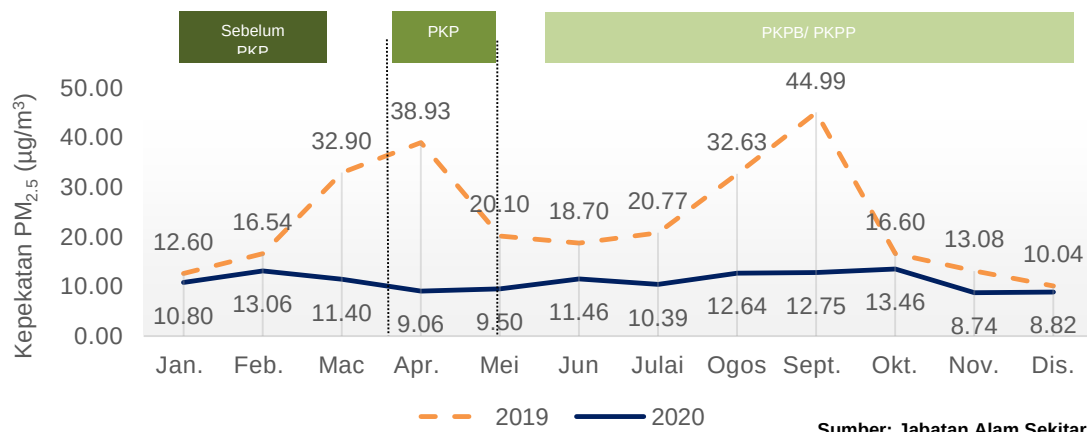
Carta 1.6: Purata bulanan kepekatan PM 2.5 di udara, Stesen Balok Baru, Pahang, 2019 dan 2020
