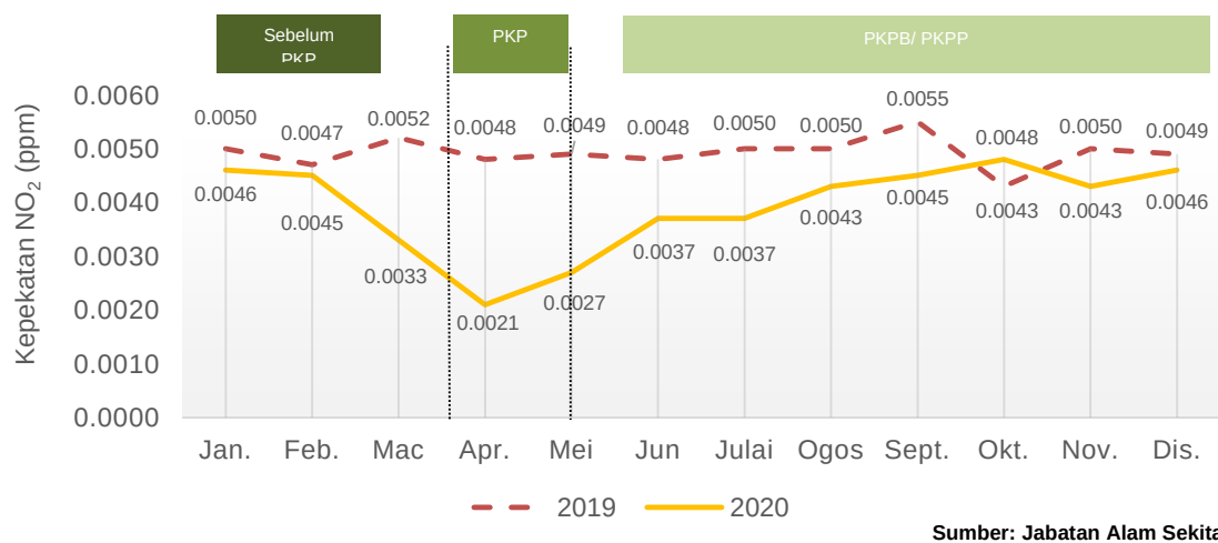
Carta 1.24: Purata bulanan kepekatan NO 2 di udara, stesen Temerloh, Pahang, 2019 dan 2020
