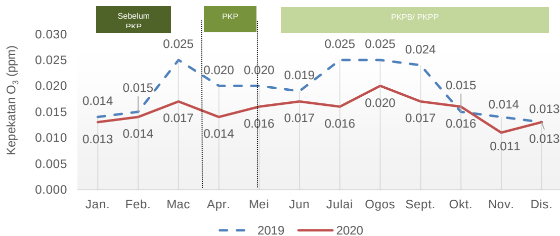
Carta 1.11: Purata bulanan kepekatan O 3 di udara, stesen Jerantut, Pahang, 2019 dan 2020
