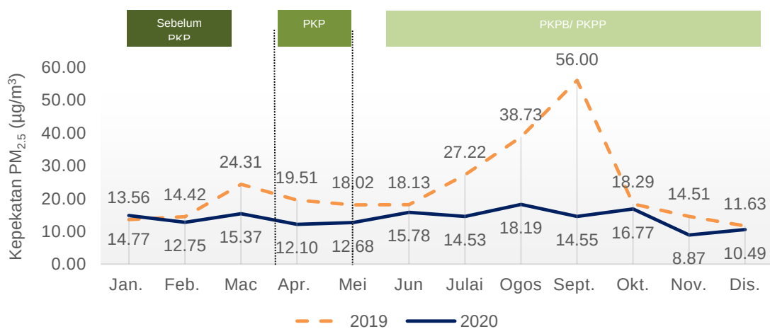
Carta 1.10: Purata bulanan kepekatan PM 2.5 di udara, stesen Temerloh, Pahang, 2019 dan 2020
