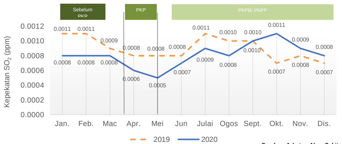
Carta 1.18: Purata bulanan kepekatan SO 2 di udara, stesen Jerantut, Pahang, 2019 dan 2020
