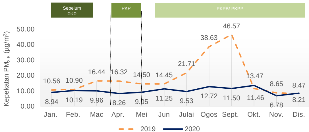
Carta 1.8: Purata bulanan kepekatan PM 2.5 di udara, stesen Kuantan, Pahang, 2019 dan 2020
