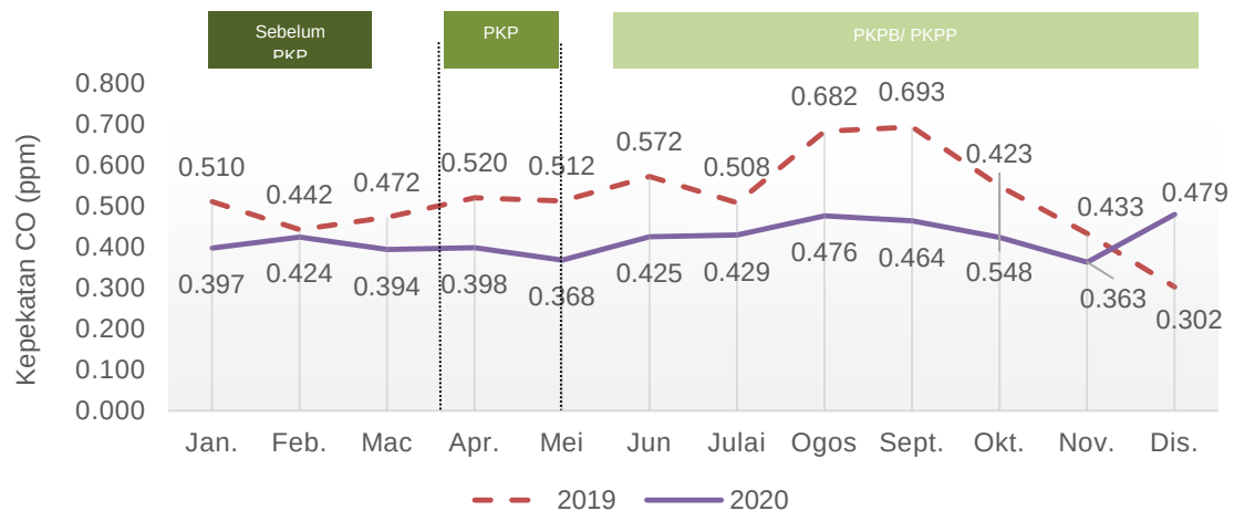
Carta 1.15: Purata bulanan kepekatan CO di udara, stesen Kuantan, Pahang, 2019 dan 2020
