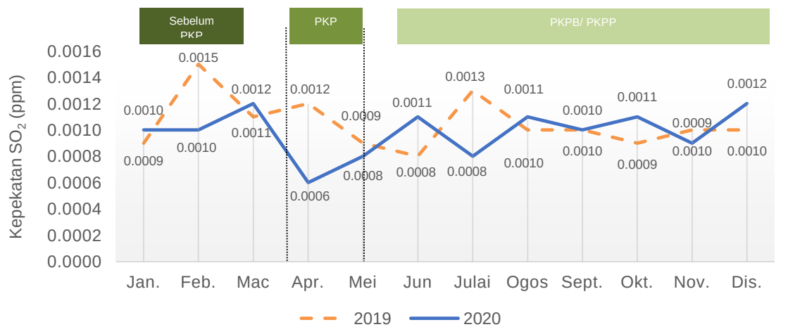
Carta 1.19: Purata bulanan kepekatan SO 2 di udara, stesen Kuantan, Pahang, 2019 dan 2020
