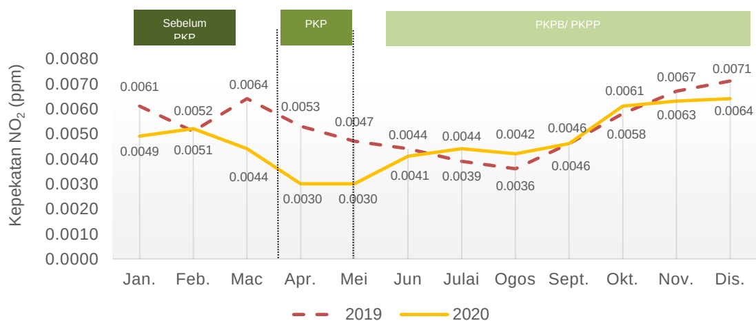
Carta 1.21: Purata bulanan kepekatan NO 2 di udara, stesen Balok Baru, Pahang, 2019 dan 2020
