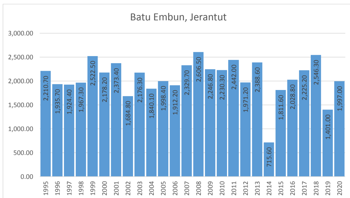
Carta1.1: Taburan hujan di stesen meteorologi Batu Embun, Jerantut, Pahang, 1995-2020
