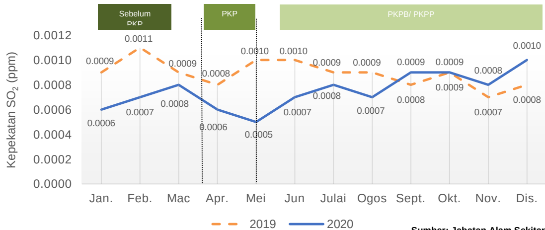
Carta 1.20: Purata bulanan kepekatan SO 2 di udara, stesen Temerloh, Pahang, 2019 dan 2020
