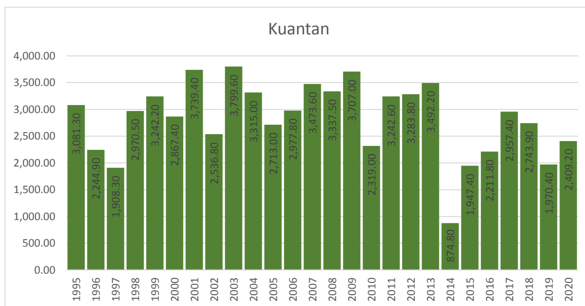
Carta1.3: Taburan hujan di stesen meteorologi Kuantan, Pahang, 1995-2020
