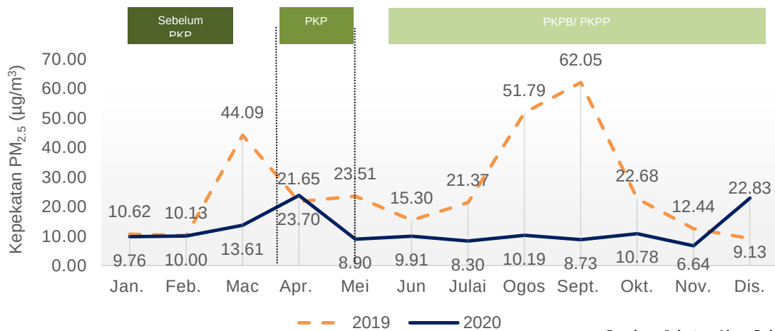
Carta 1.9: Purata bulanan kepekatan PM 2.5 di udara, stesen Rompin, Pahang, 2019 dan 2020
