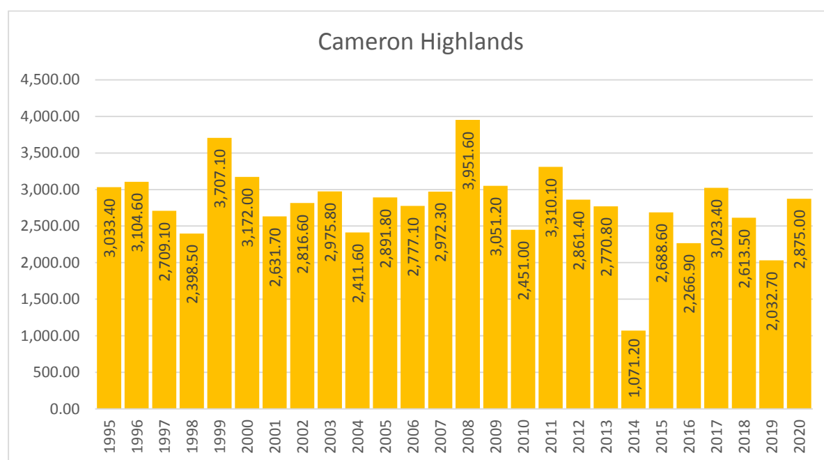
Carta 1.2: Taburan hujan di stesen meteorologi Cameron Highlands, Pahang, 1995-2020
