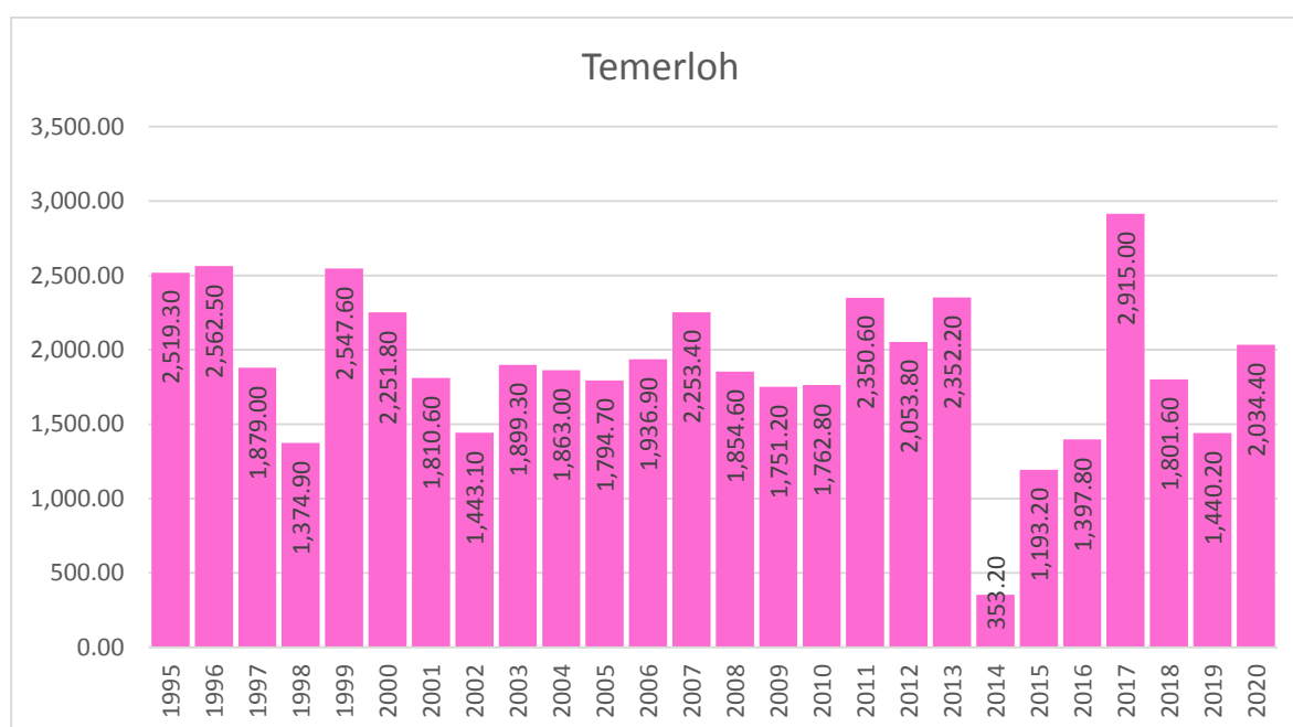
Carta1.5: Taburan hujan di stesen meteorologi Temerloh, Pahang, 1995-2020
