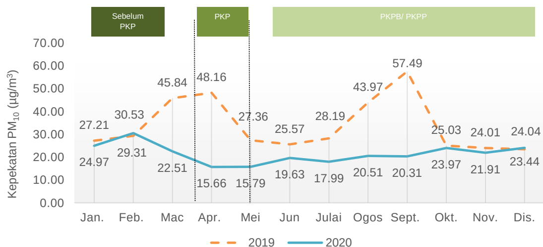
Carta 1.1: Purata bulanan kepekatan PM_{10} di udara, stesen Balok Baru, Pahang, 2019 dan 2020
