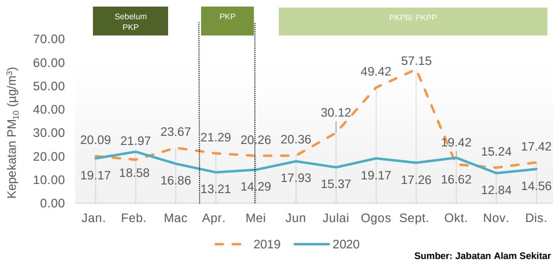
Carta 1.3: Purata bulanan kepekatan PM 10 di udara, stesen Kuantan, Pahang, 2019 dan 2020
