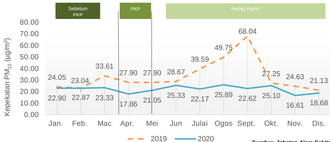
Carta 1.5: Purata bulanan kepekatan PM 10 di udara, stesen Temerloh, Pahang, 2019 dan 2020
