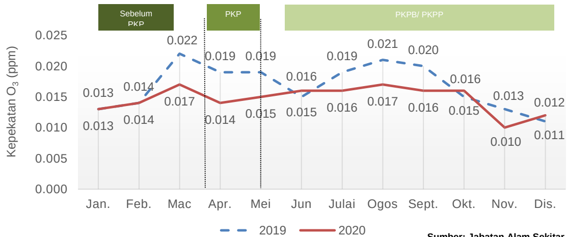
Carta 1.13: Purata bulanan kepekatan O 3 di udara, stesen Temerloh, Pahang, 2019 dan 2020
