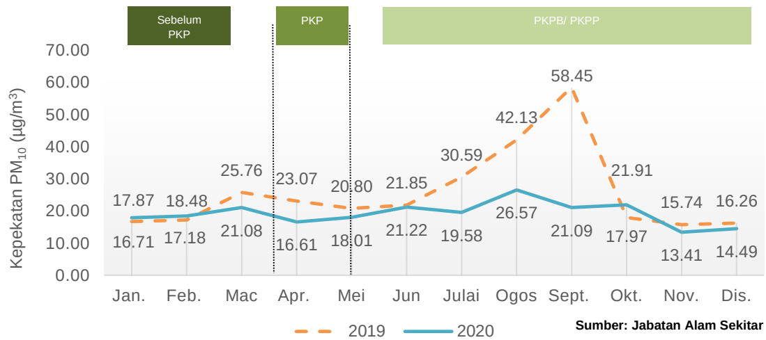
Carta 1.2: Purata bulanan kepekatan PM 10 di udara, stesen Jerantut, Pahang, 2019 dan 2020
