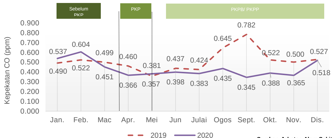
Carta 1.16: Purata bulanan kepekatan CO di udara, stesen Temerloh, Pahang, 2019 dan 2020
