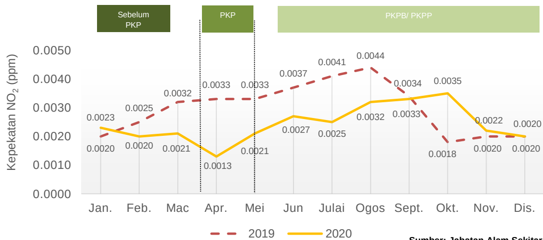
Carta 1.22: Purata bulanan kepekatan NO 2 di udara, stesen Jerantut, Pahang, 2019 dan 2020
