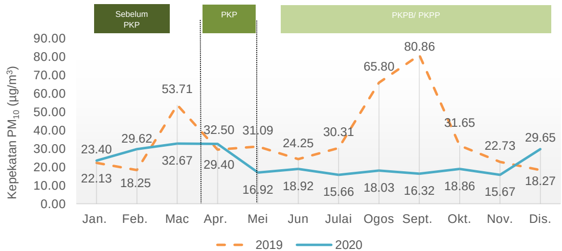
Carta 1.4: Purata bulanan kepekatan PM 10 di udara, stesen Rompin, Pahang, 2019 dan 2020
