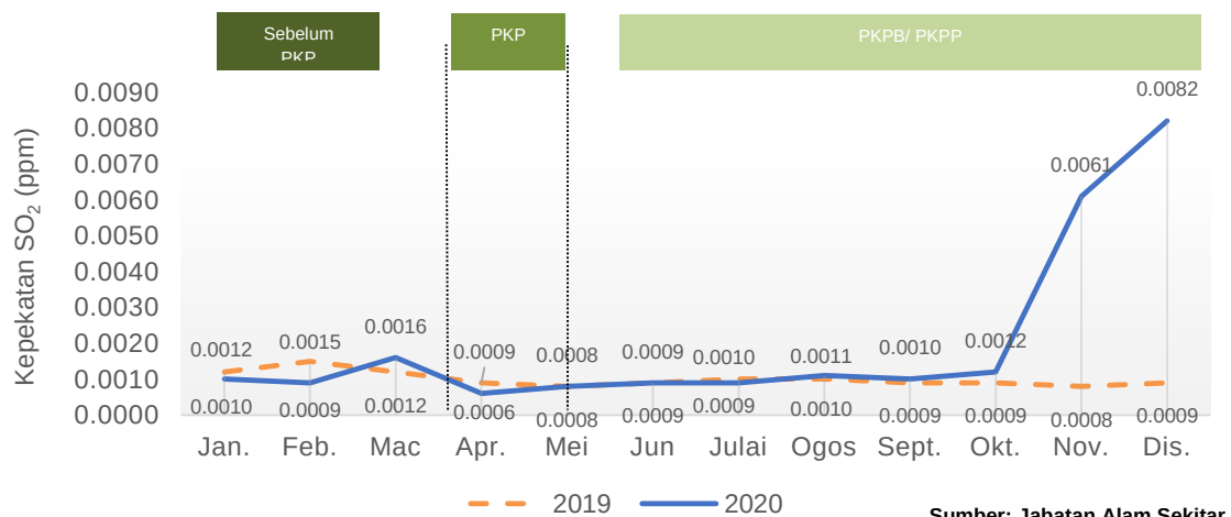
Carta 1.17: Purata bulanan kepekatan SO 2 di udara, stesen Balok Baru, Pahang, 2019 dan 2020
