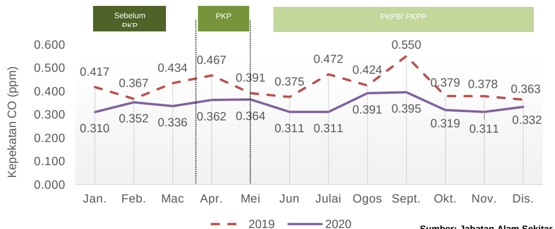
Carta 1.14: Purata bulanan kepekatan CO di udara, stesen Jerantut, Pahang, 2019 dan 2020
