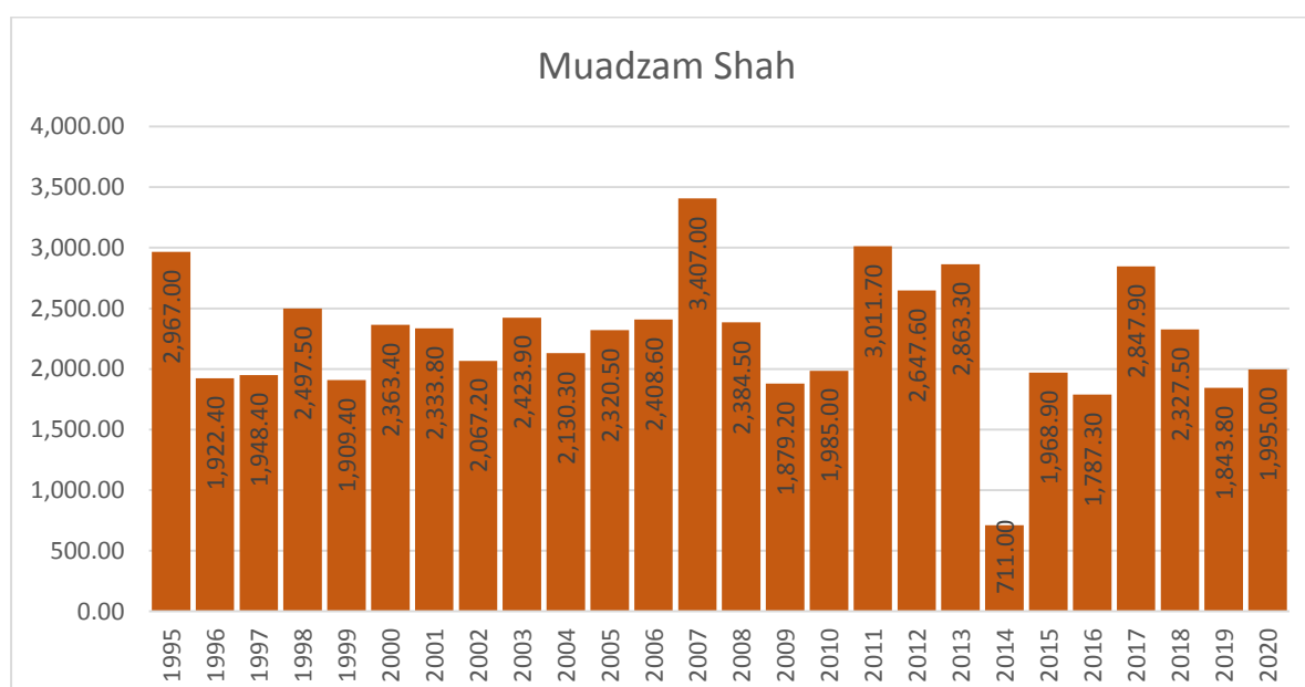
Carta1.4: Taburan hujan di stesen meteorologi Muadzam Shah, Pahang, 1995-2020
