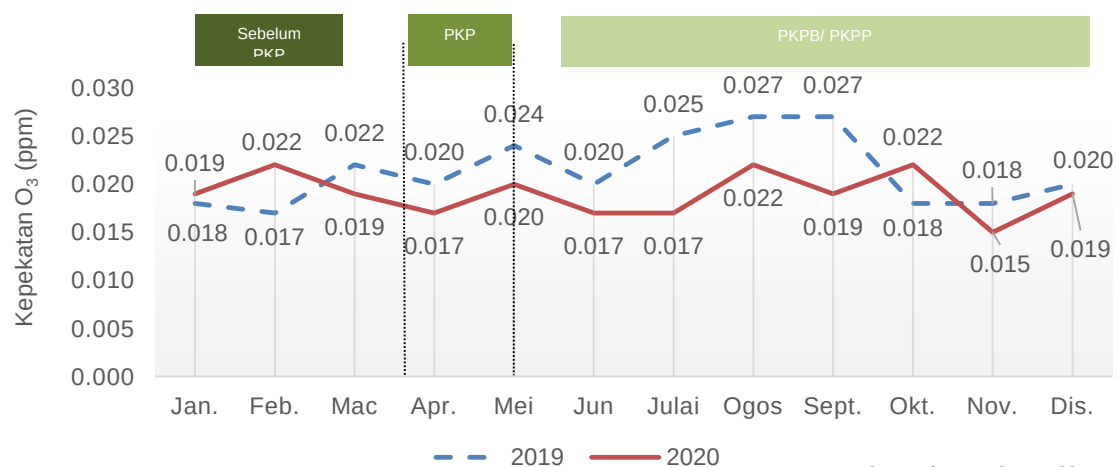
Carta 1.12: Purata bulanan kepekatan O 3 di udara, stesen Kuantan, Pahang, 2019 dan 2020
