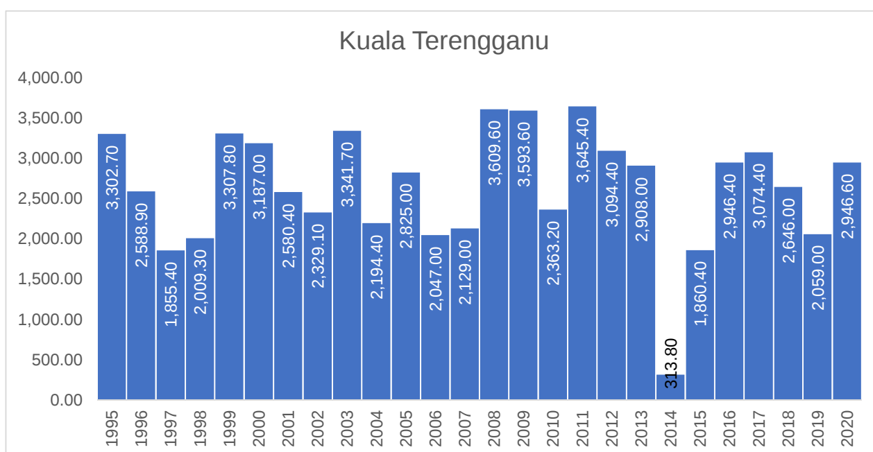
Carta1.1: Taburan hujan di stesen meteorologi Kuala Terengganu, Terengganu, 1995-2020
