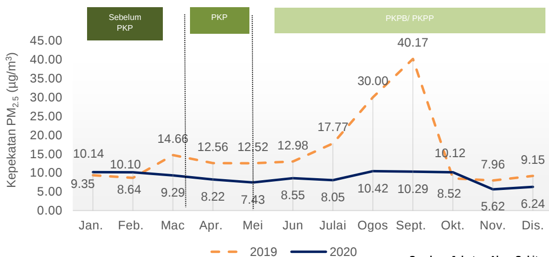
Carta 1.8: Purata bulanan kepekatan PM 2.5 di udara, stesen Paka, Terengganu, 2019 dan 2020
