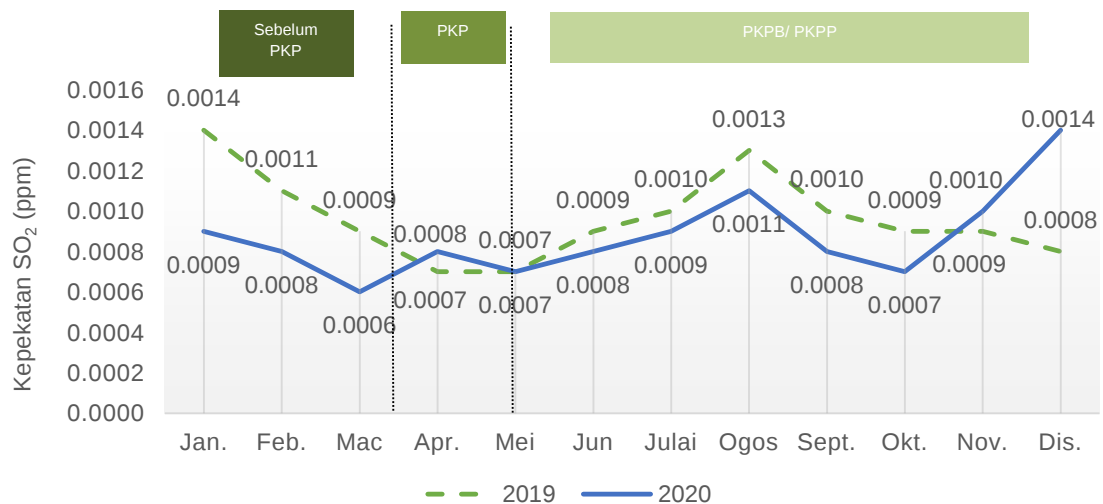
Carta 1.14: Purata bulanan kepekatan SO 2 di udara, stesen Kemaman, Terengganu, 2019 dan 2020
