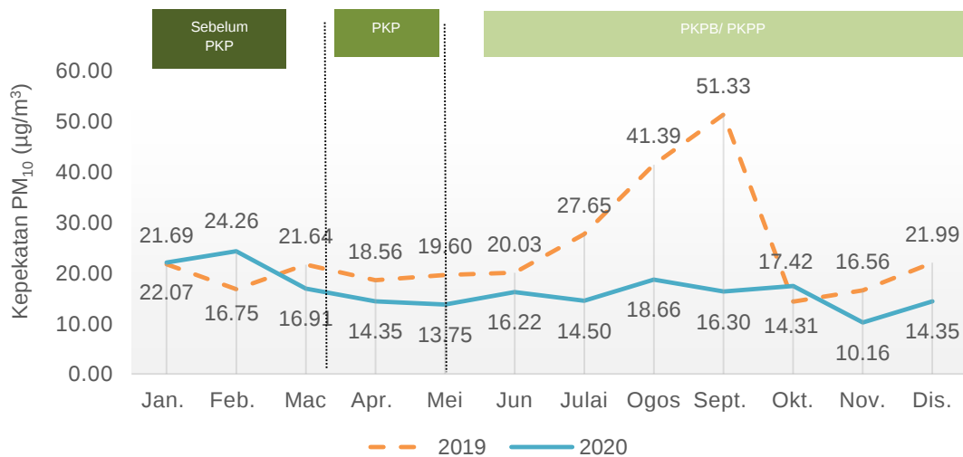
Carta 1.4: Purata bulanan kepekatan PM 10 di udara, stesen Paka, Terengganu, 2019 dan 2020
