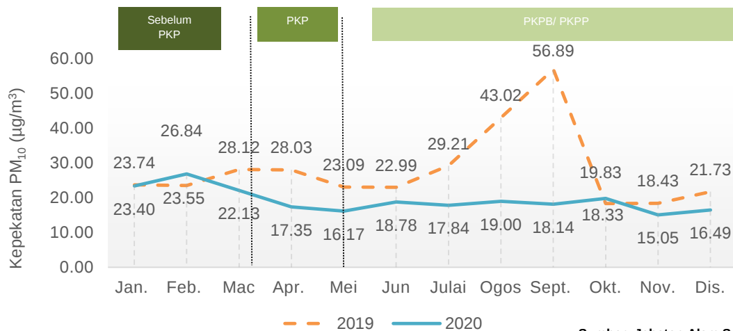
Carta 1.2: Purata bulanan kepekatan PM 10 di udara, stesen Kemaman, Terengganu, 2019 dan 2020
