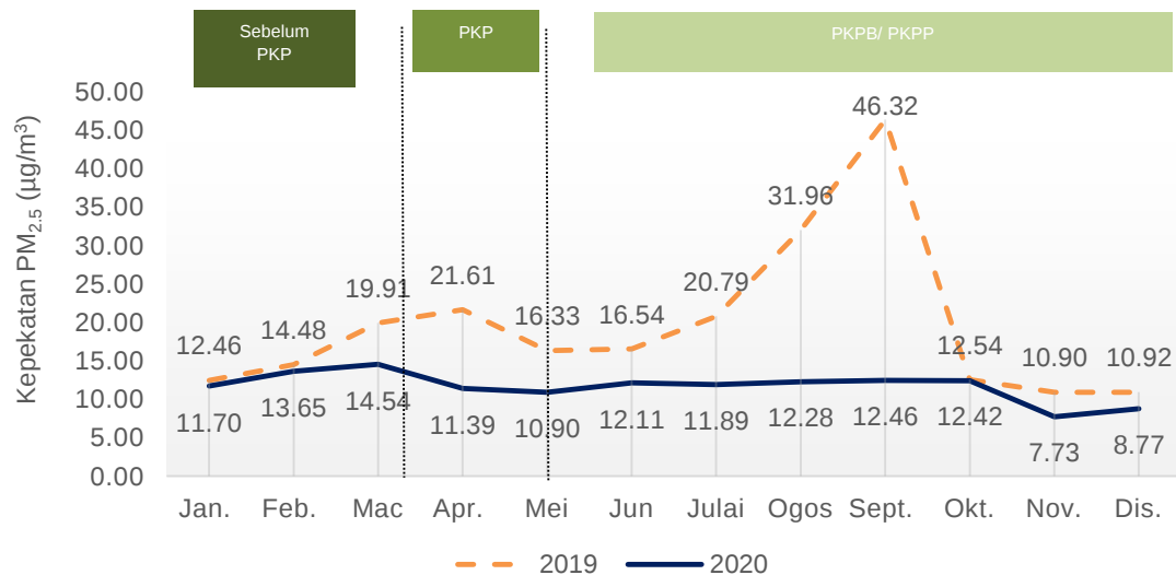
Carta 1.6: Purata bulanan kepekatan PM_{2.5} di udara, stesen Kemaman, Terengganu, 2019 dan 2020
