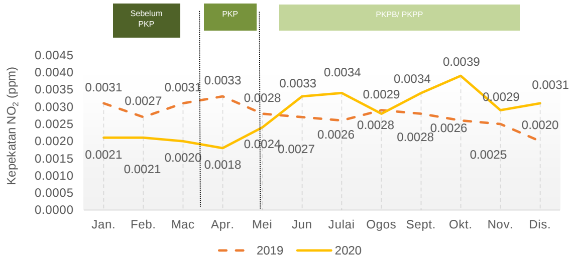
Carta 1.18: Purata bulanan kepekatan NO 2 di udara, stesen Kemaman, Terengganu, 2019 dan 2020
