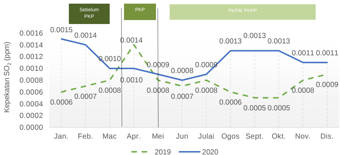
Carta 1.15: Purata bulanan kepekatan SO 2 di udara, stesen Kuala Terengganu, Terengganu, 2019 dan 2020
