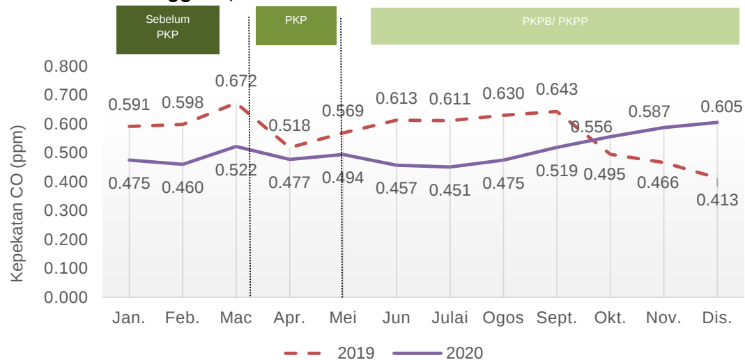
Carta 1.12: Purata bulanan kepekatan CO di udara, stesen Kuala Terengganu, Terengganu, 2019 dan 2020
