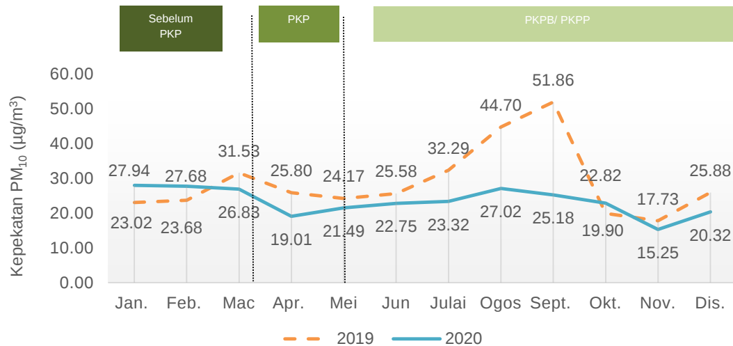
Carta 1.3: Purata bulanan kepekatan PM 10 di udara, stesen Kuala Terengganu, Terengganu, 2019 dan 2020
