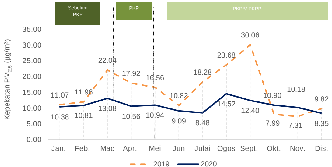
Carta 1.5: Purata bulanan kepekatan PM_{2.5} di udara, stesen Besut, Terengganu, 2019 dan 2020
