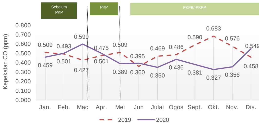
Carta 1.11: Purata bulanan kepekatan CO di udara, stesen Besut Terengganu, 2019 dan 2020
