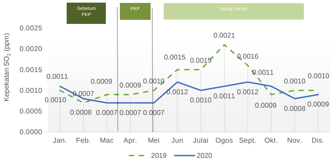
Carta 1.16: Purata bulanan kepekatan SO 2 di udara, stesen Paka, Terengganu, 2019 dan 2020
