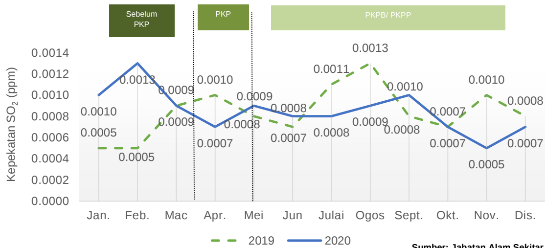
Carta 1.13: Purata bulanan kepekatan SO 2 di udara, stesen Besut Terengganu, 2019 dan 2020
