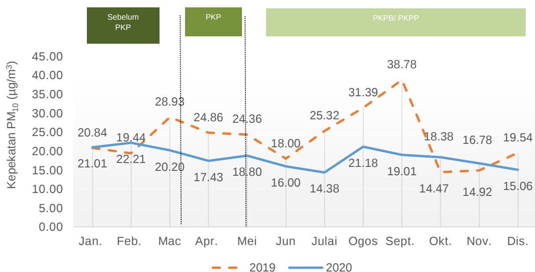
Carta 1.1: Purata bulanan kepekatan PM_{10} di udara, stesen Besut, Terengganu, 2019 dan 2020
