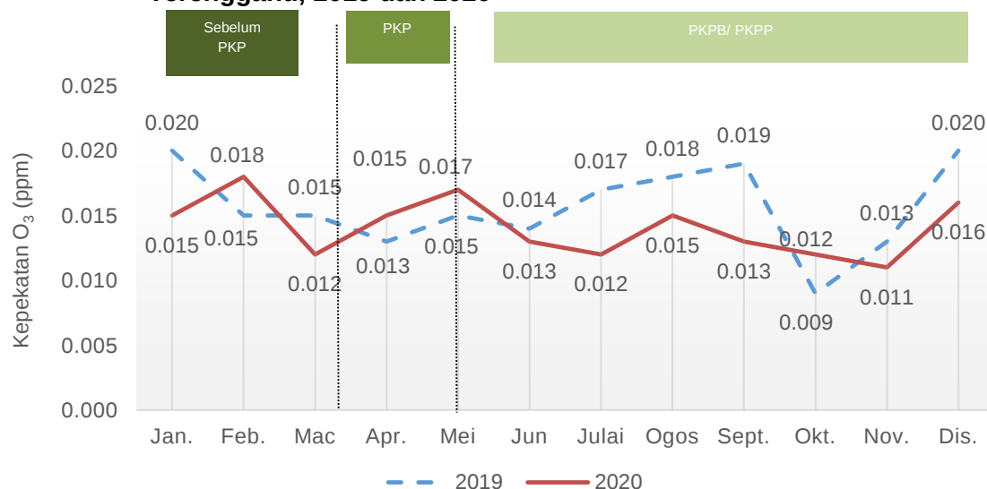
Carta 1.10: Purata bulanan kepekatan O 3 di udara, stesen Kuala Terengganu, Terengganu, 2019 dan 2020
