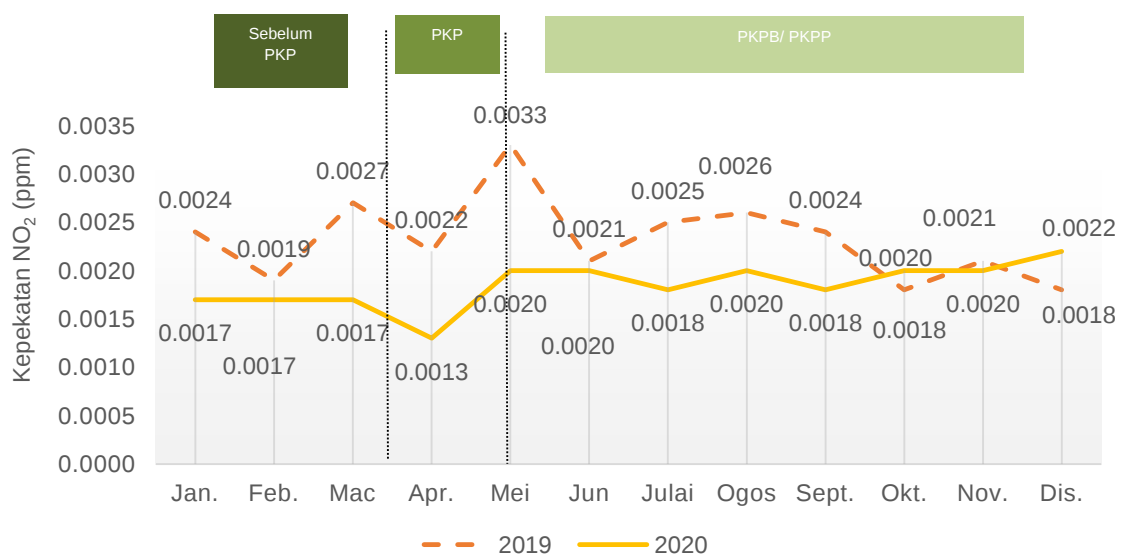
Carta 1.17: Purata bulanan kepekatan NO 2 di udara, stesen Besut, Terengganu, 2019 dan 2020
