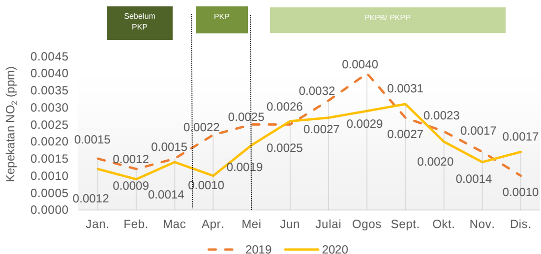
Carta 1.20: Purata bulanan kepekatan NO 2 di udara, stesen Paka, Terengganu, 2019 dan 2020
