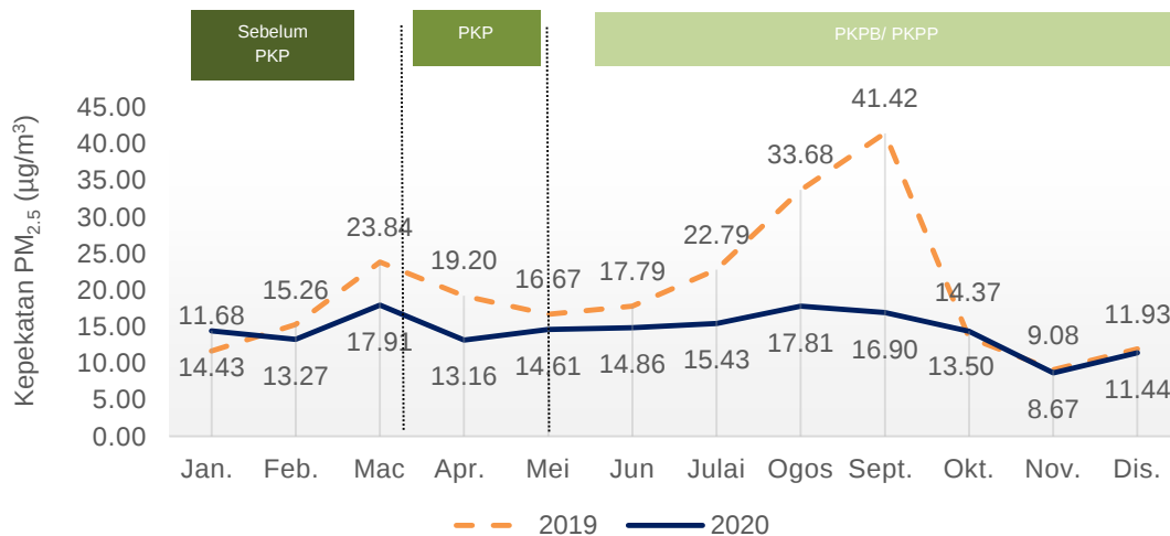
Carta 1.7: Purata bulanan kepekatan PM 2.5 di udara, stesen Kuala Terengganu, Terengganu, 2019 dan 2020
