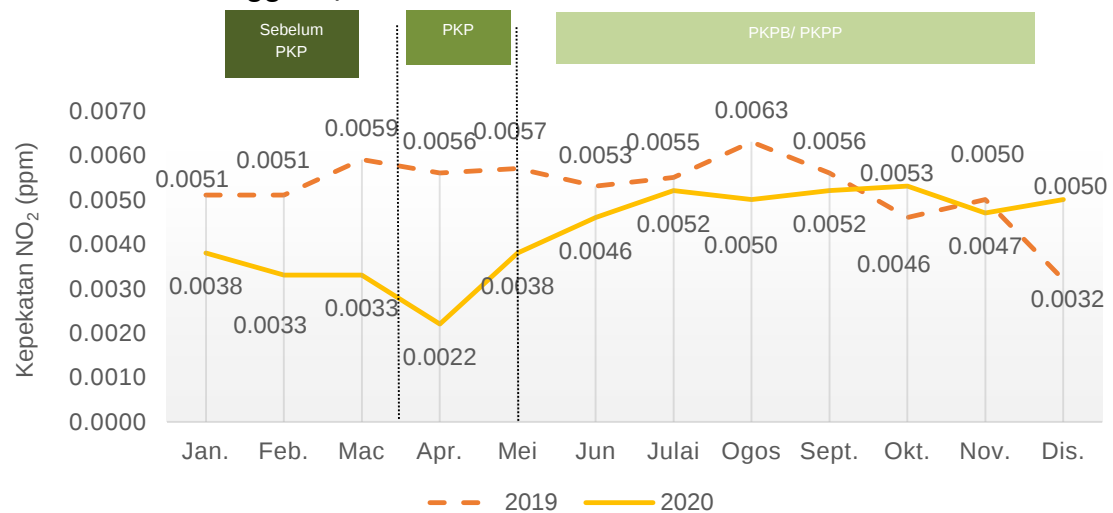
Carta 1.19: Purata bulanan kepekatan NO 2 di udara, stesen Kuala Terengganu, Terengganu, 2019 dan 2020
