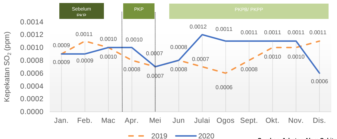
Carta 1.16: Purata bulanan kepekatan SO 2 di udara, stesen Kulim, Kedah, 2019 dan 2020
