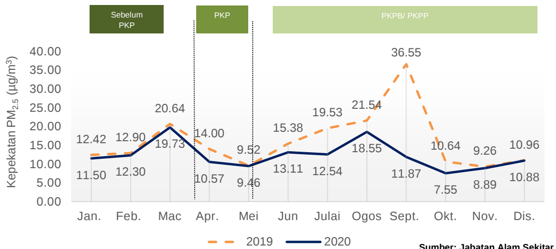
Carta 1.5: Purata bulanan kepekatan PM_{2.5} di udara, stesen Alor Setar, 2019 dan 2020
