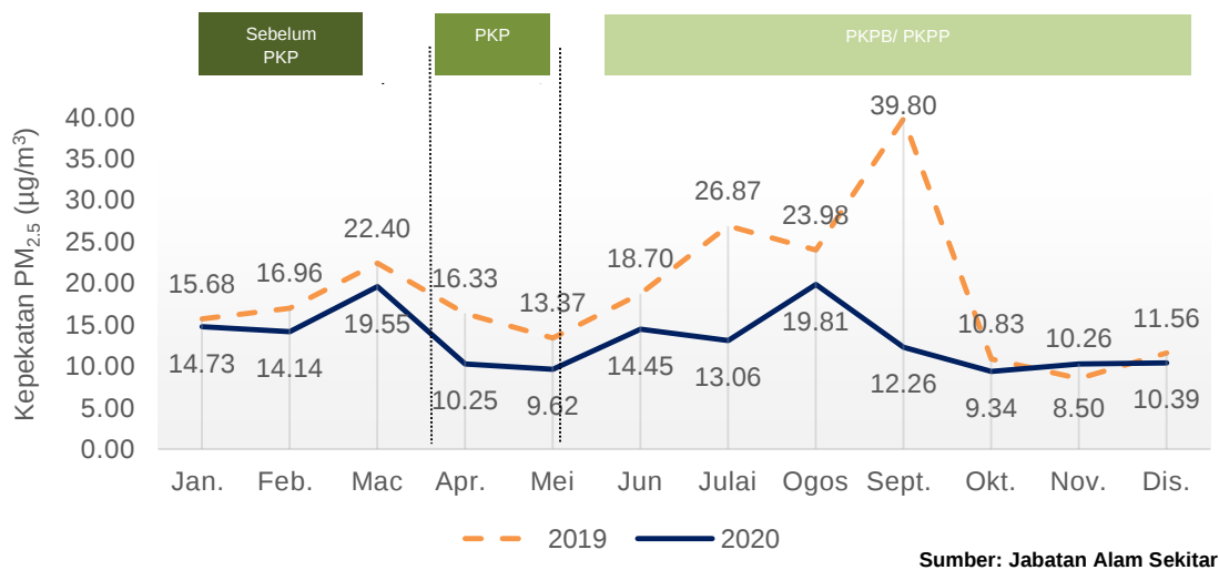
Carta 1.6: Purata bulanan kepekatan PM_{2.5} di udara, stesen Kulim, Kedah, 2019 dan 2020
