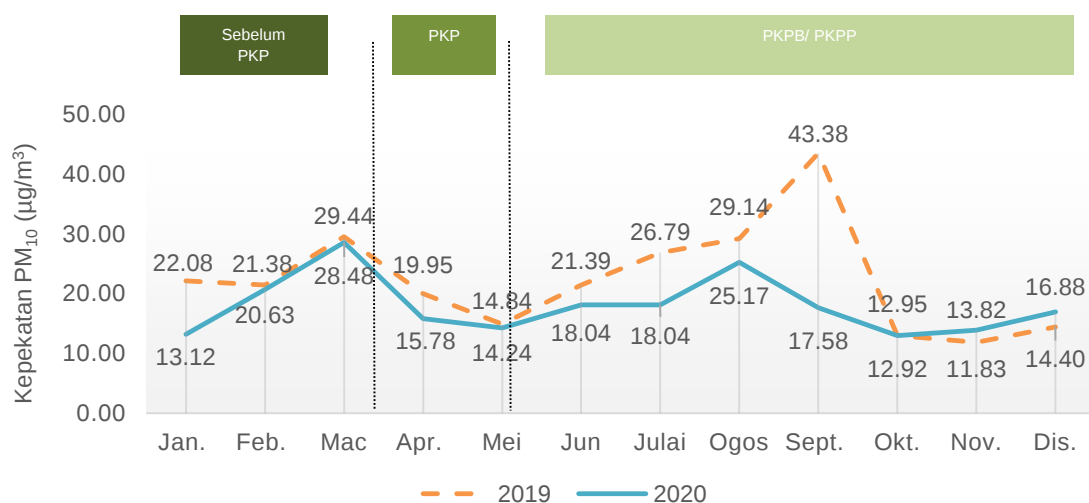
Carta 1.1: Purata bulanan kepekatan PM_{10} di udara, stesen Alor Setar, Kedah, 2019 dan 2020
