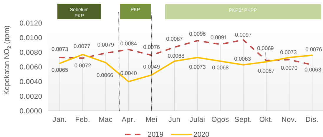
Carta 1.22: Purata bulanan kepekatan NO 2 di udara, stesen Sungai Petani, Kedah, 2019 dan 2020
