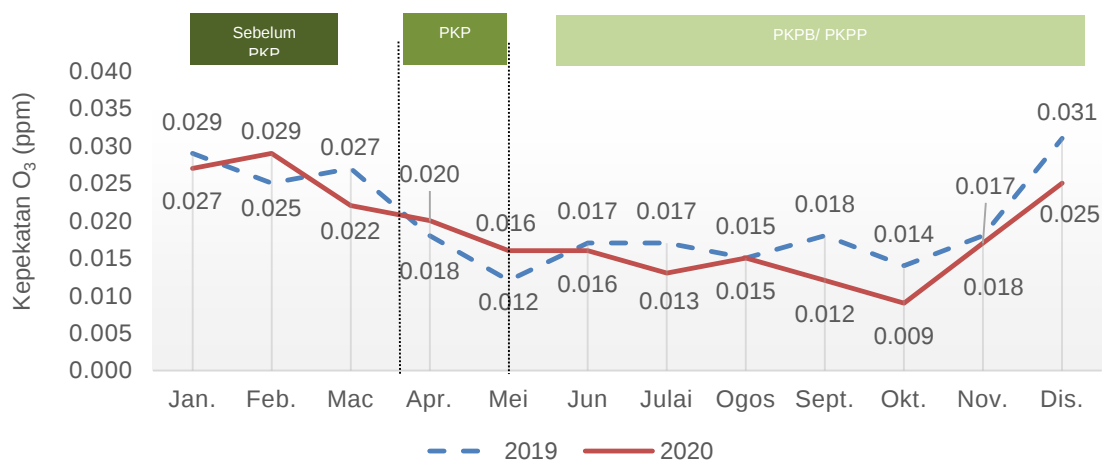
Carta 1.10: Purata bulanan kepekatan O 3 di udara, stesen Langkawi, Kedah, 2019 dan 2020
