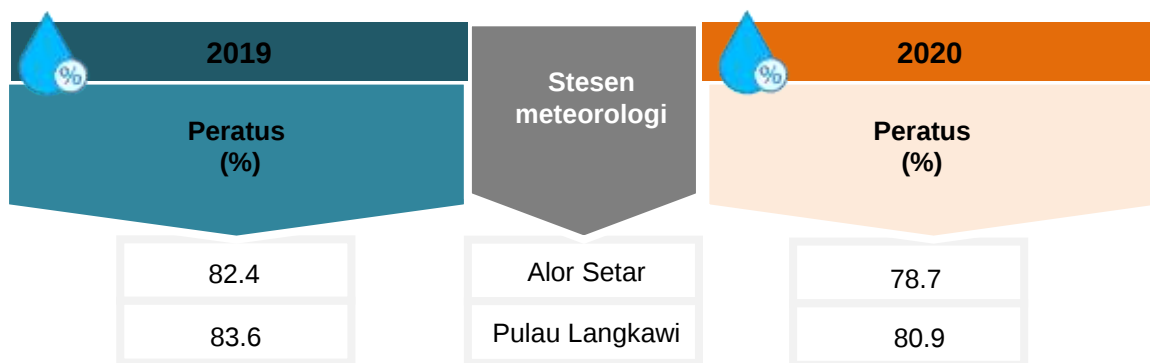
Paparan 1.3: Purata kelembapan relatif di stesen meteorologi, Kedah, 2019 dan 2020
