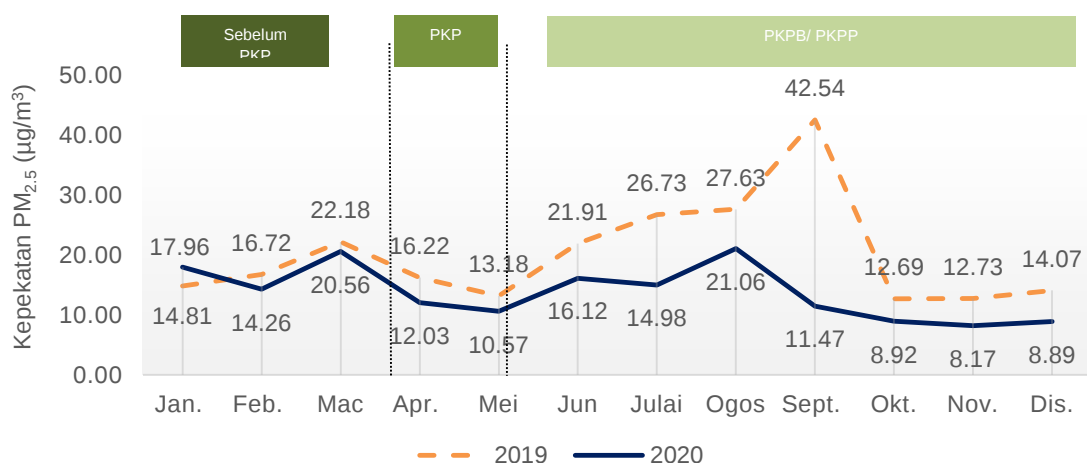
Carta 1.8: Purata bulanan kepekatan PM 2.5 di udara, stesen Sungai Petani, Kedah, 2019 dan 2020
