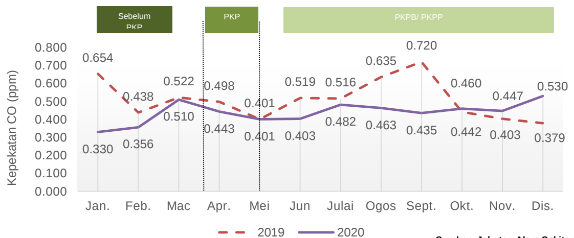
Carta 1.12: Purata bulanan kepekatan CO di udara, stesen Alor Setar, Kedah, 2019 dan 2020
