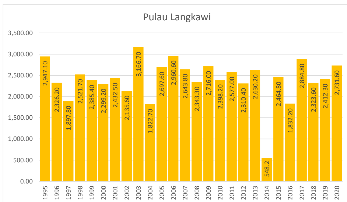
Carta 1.2: Taburan hujan di stesen meteorologi Pulau Langkawi, Kedah, 1995 - 2020
