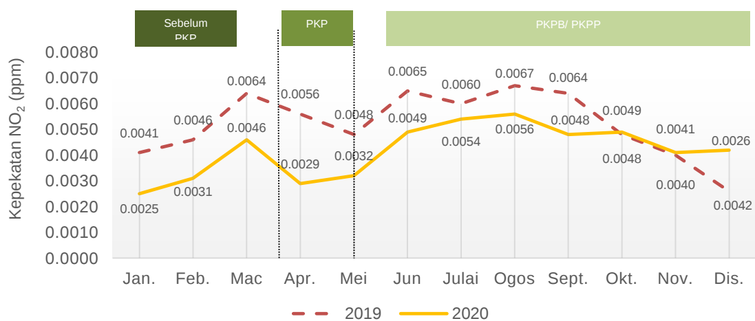
Carta 1.19: Purata bulanan kepekatan NO 2 di udara, stesen Alor Setar, Kedah, 2019 dan 2020
