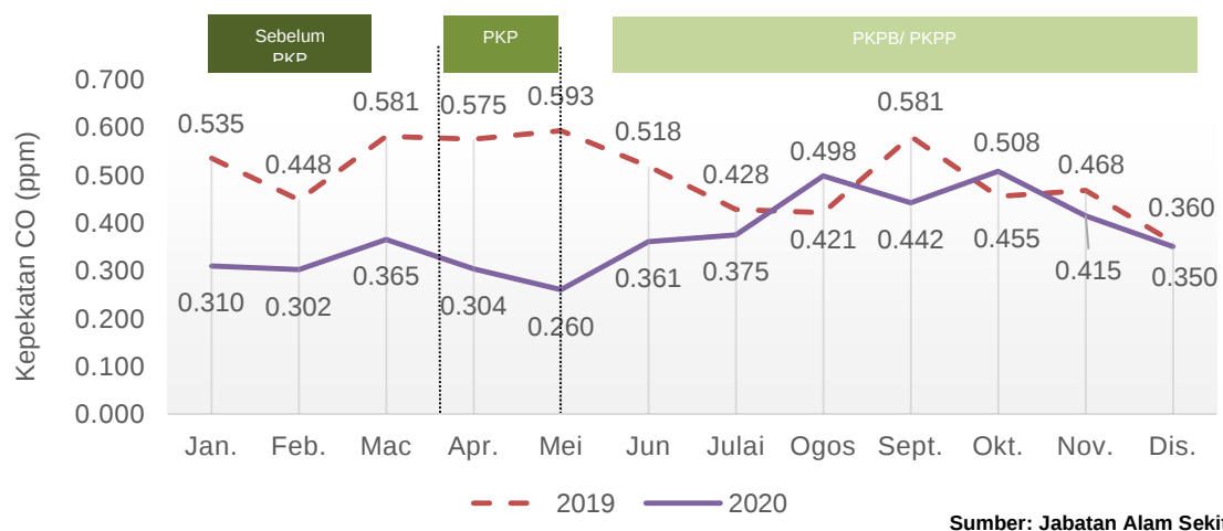
Carta 1.13: Purata bulanan kepekatan CO di udara, stesen Langkawi, Kedah, 2019 dan 2020
