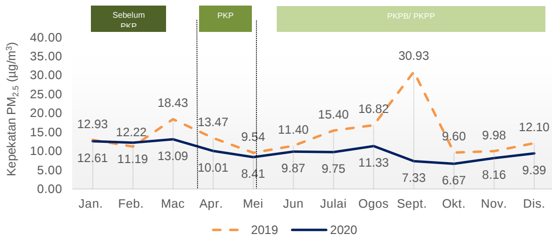
Carta 1.7: Purata bulanan kepekatan PM 2.5 di udara, stesen Langkawi, Kedah, 2019 dan 2020
