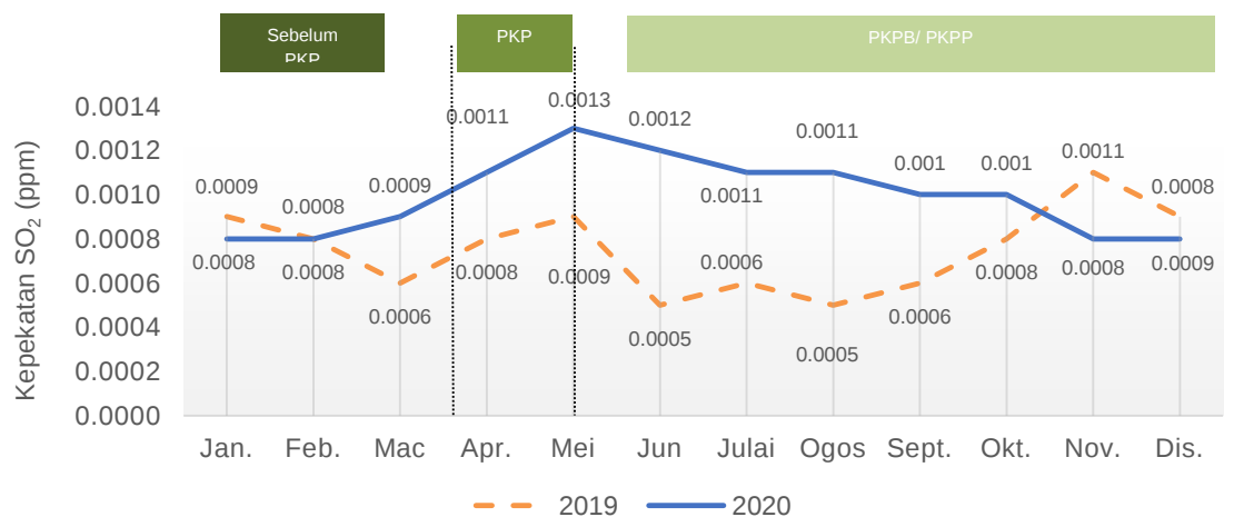
Carta 1.17: Purata bulanan kepekatan SO 2 di udara, stesen Langkawi, Kedah, 2019 dan 2020
