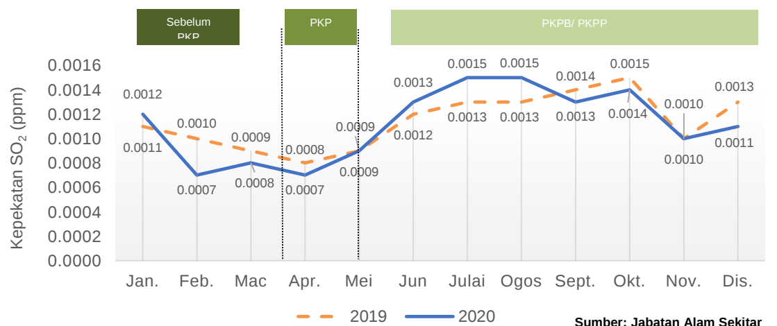
Carta 1.18: Purata bulanan kepekatan SO 2 di udara, stesen Sungai Petani, Kedah, 2019 dan 2020
