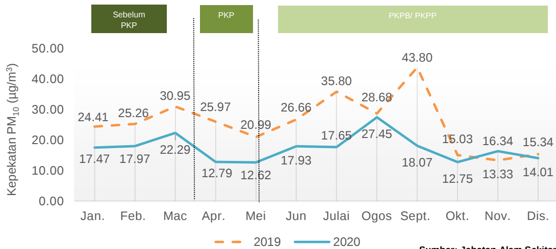
Carta 1.2: Purata bulanan kepekatan PM 10 di udara, stesen Kulim, Kedah, 2019 dan 2020
