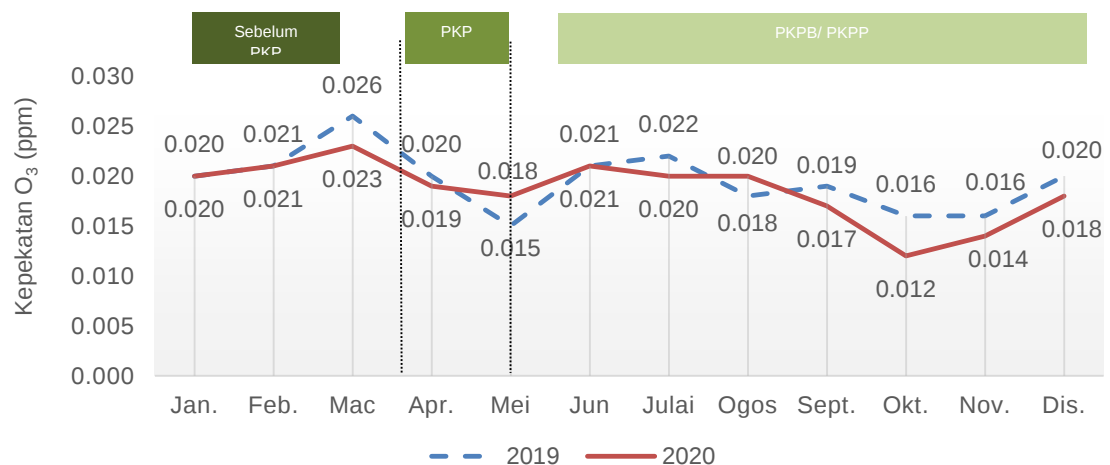
Carta 1.11: Purata bulanan kepekatan O 3 di udara, stesen Sungai Petani, Kedah, 2019 dan 2020
