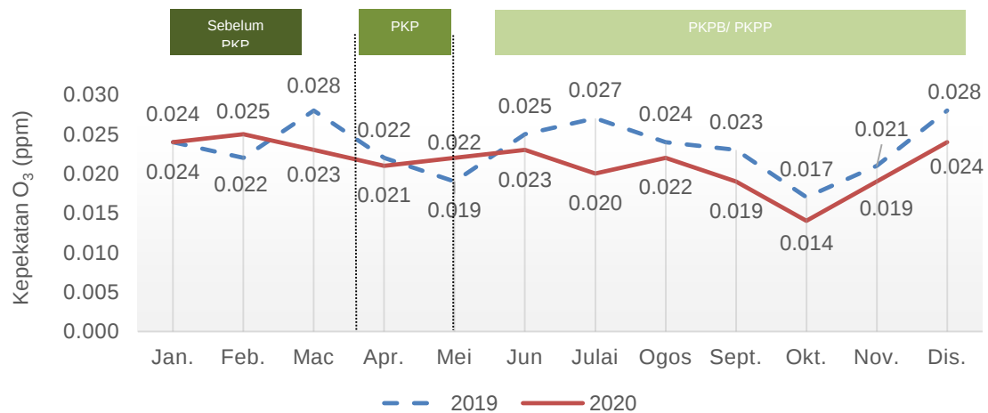
Carta 1.9: Purata bulanan kepekatan O 3 di udara, stesen Alor Setar, Kedah, 2019 dan 2020
