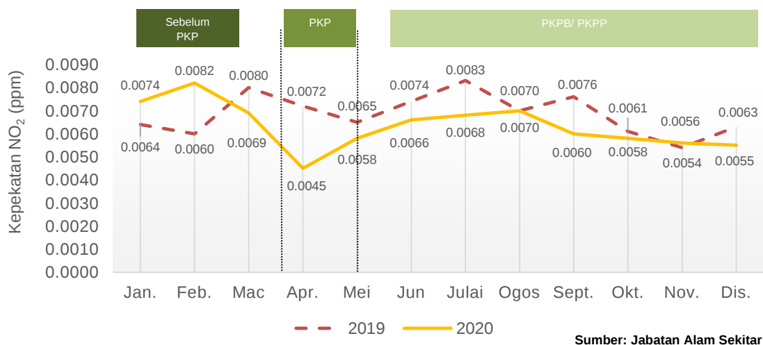
Carta 1.20: Purata bulanan kepekatan NO 2 di udara, stesen Kulim, Kedah, 2019 dan 2020
