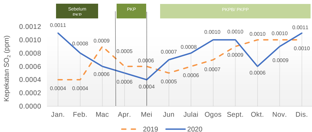
Carta 1.15: Purata bulanan kepekatan SO 2 di udara, stesen Alor Setar, Kedah, 2019 dan 2020
