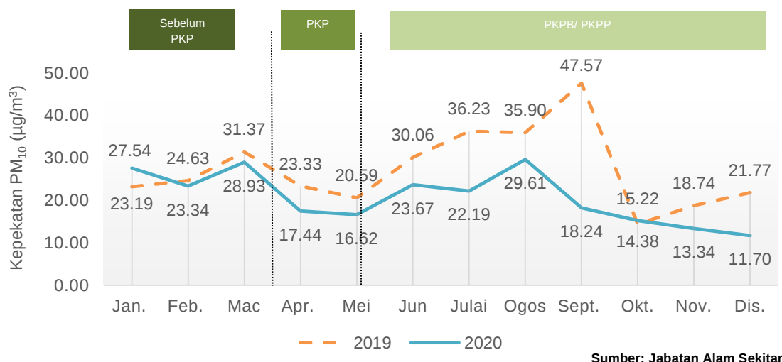
Carta 1.4: Purata bulanan kepekatan PM 10 di udara, stesen Sungai Petani, Kedah, 2019 dan 2020
