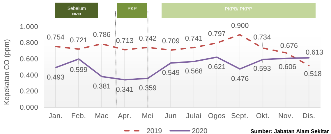
Carta 1.14: Purata bulanan kepekatan CO di udara, stesen Sungai Petani, Kedah, 2019 dan 2020
