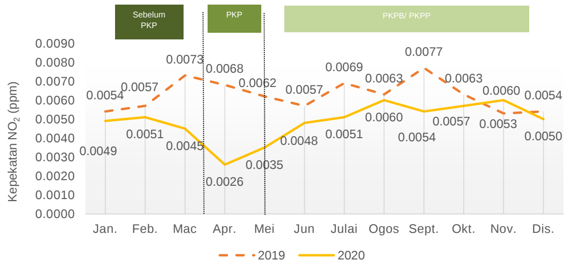
Carta 1.25: Purata bulanan kepekatan NO 2 di udara, stesen Tanjung Malim, Perak, 2019 dan 2020
