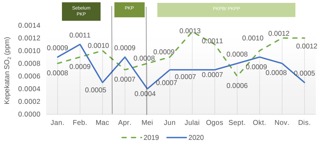
Carta 1.19: Purata bulanan kepekatan SO 2 di udara, stesen Pegoh, Ipoh, Perak, 2019 dan 2020
