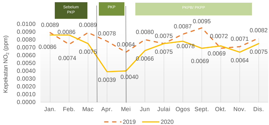
Carta 1.24: Purata bulanan kepekatan NO 2 di udara, stesen Taiping, Perak, 2019 dan 2020
