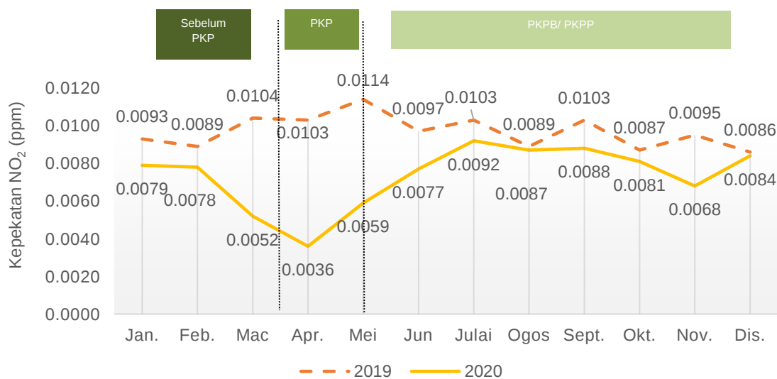
Carta 1.23: Purata bulanan kepekatan NO 2 di udara, stesen Pegoh, Ipoh, Perak, 2019 dan 2020
