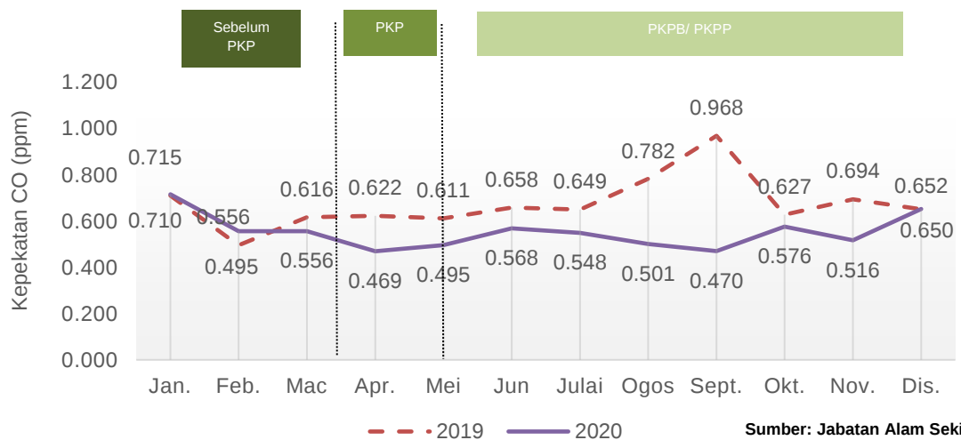
Carta 1.18: Purata bulanan kepekatan CO di udara, stesen Tasek, Ipoh, Perak, 2019 dan 2020
