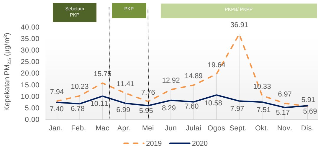
Carta 1.9: Purata bulanan kepekatan PM 2.5 di udara, stesen Tanjung Malim, Perak, 2019 dan 2020
