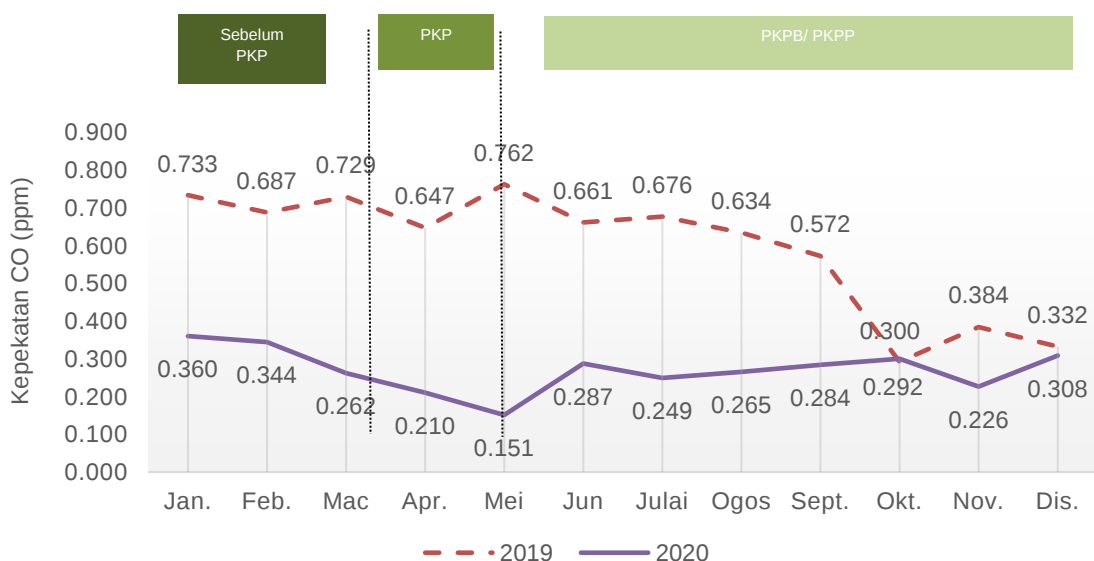
Carta 1.16: Purata bulanan kepekatan CO di udara, stesen Taiping, Perak, 2019 dan 2020
