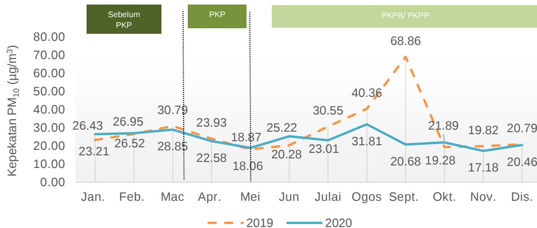
Carta 1.2: Purata bulanan kepekatan PM 10 di udara, stesen Seri Manjung, Perak, 2019 dan 2020
