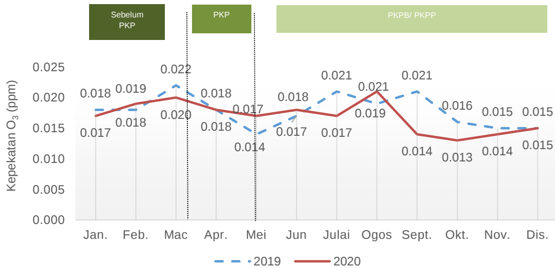
Carta 1.12: Purata bulanan kepekatan O 3 di udara, stesen Taiping, Perak, 2019 dan 2020
