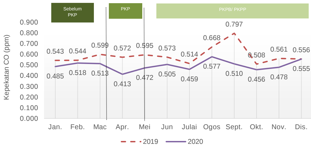
Carta 1.17: Purata bulanan kepekatan CO di udara, stesen Tanjung Malim, Perak, 2019 dan 2020
