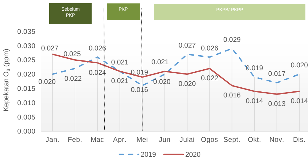
Carta 1.11: Purata bulanan kepekatan O 3 di udara, stesen Pegoh, Ipoh, Perak, 2019 dan 2020
