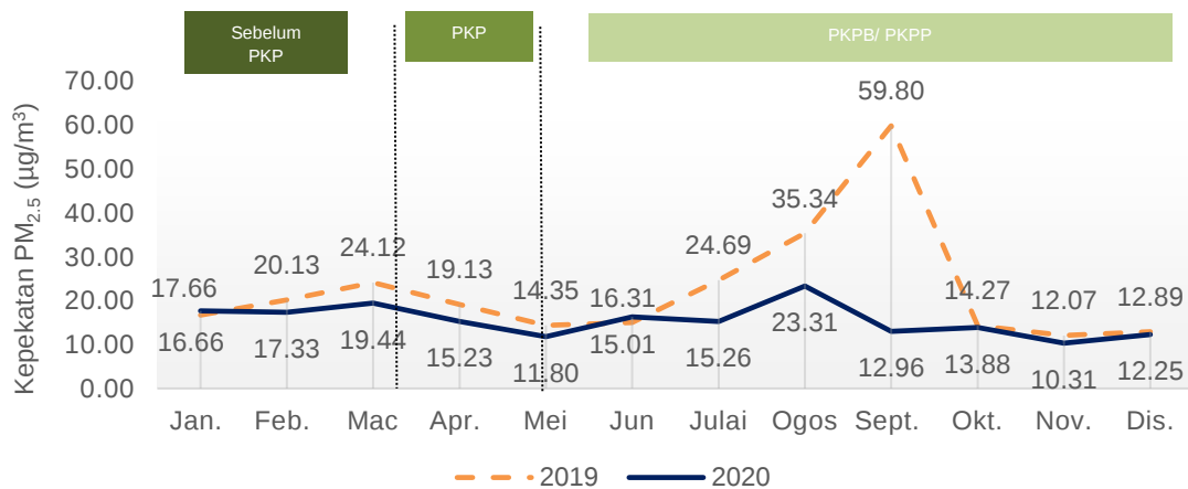
Carta 1.7: Purata bulanan kepekatan PM 2.5 di udara, stesen Seri Manjung, Perak, 2019 dan 2020
