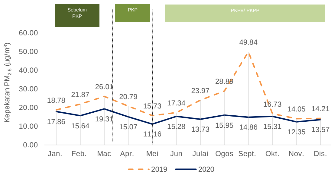
Carta 1.6: Purata bulanan kepekatan PM 2.5 di udara, stesen Pegoh, Ipoh, Perak, 2019 dan 2020
