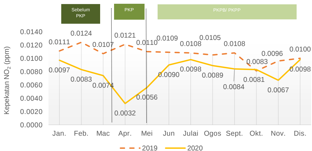
Carta 1.26: Purata bulanan kepekatan NO 2 di udara, stesen Tasek, Ipoh, Perak, 2019 dan 2020
