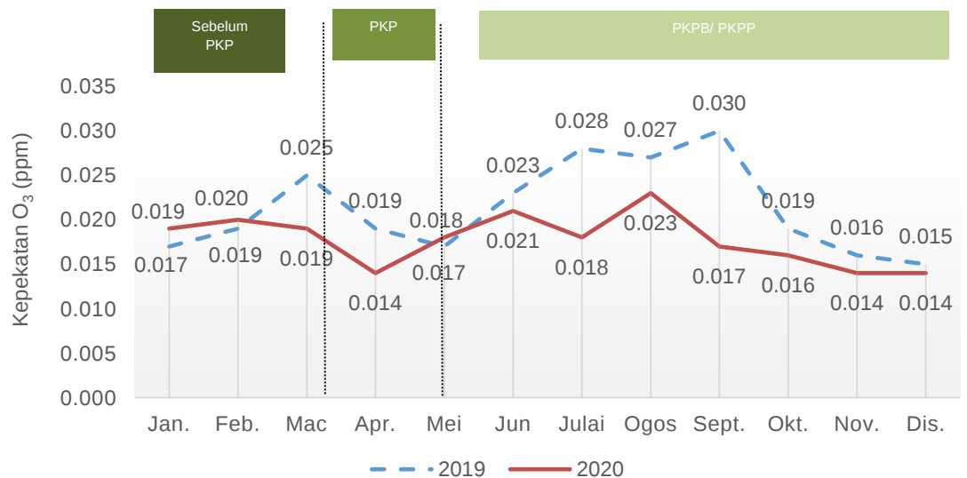
Carta 1.13: Purata bulanan kepekatan O 3 di udara, stesen Tanjung Malim, Perak, 2019 dan 2020
