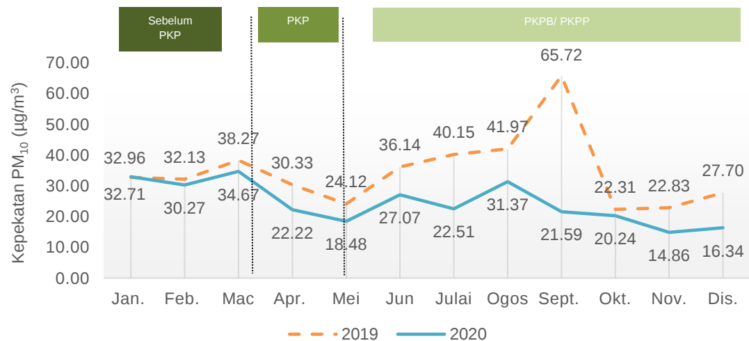
Carta 1.3: Purata bulanan kepekatan PM 10 di udara, stesen Taiping, Perak, 2019 dan 2020
