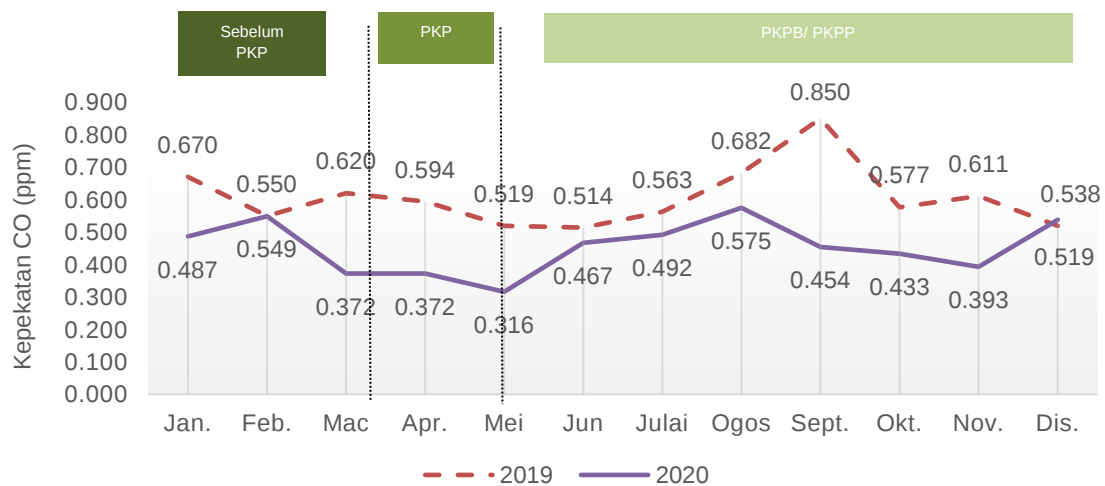
Carta 1.15: Purata bulanan kepekatan CO di udara, stesen Pegoh, Ipoh, Perak, 2019 dan 2020
