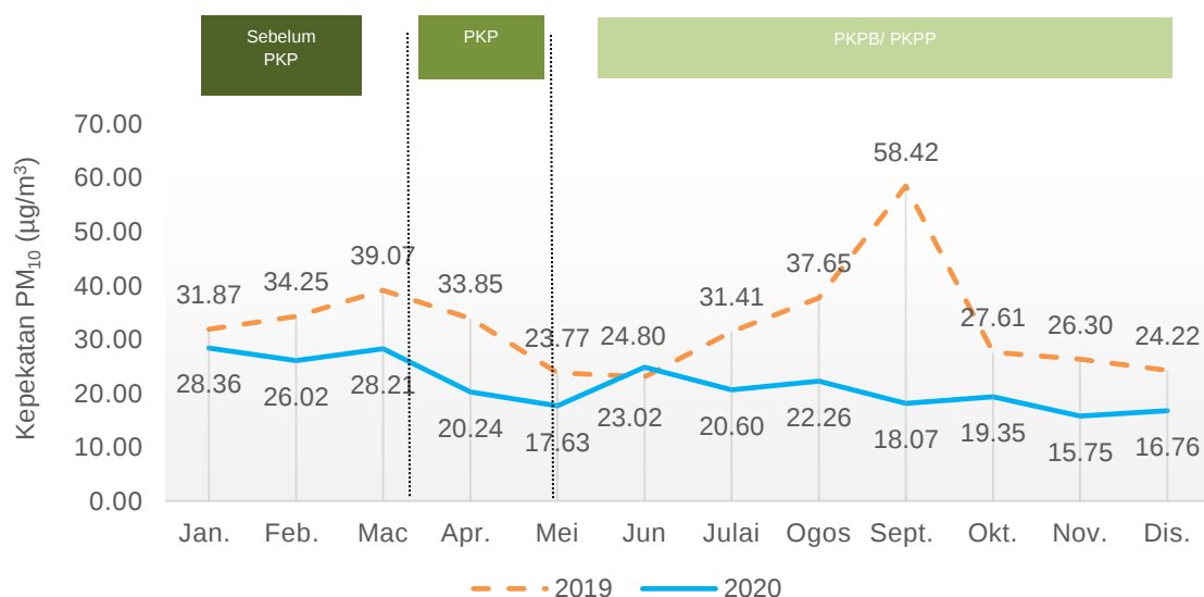
Carta 1.1: Purata bulanan kepekatan PM_{10} di udara, stesen Pegoh, Ipoh, Perak, 2019 dan 2020
