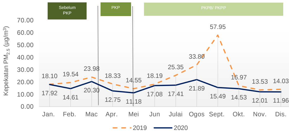
Carta 1.10: Purata bulanan kepekatan PM 2.5 di udara, stesen Tasek, Ipoh, Perak, 2019 dan 2020
