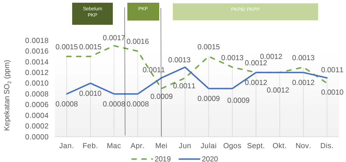
Carta 1.22: Purata bulanan kepekatan SO 2 di udara, stesen Tasek, Ipoh, Perak, 2019 dan 2020
