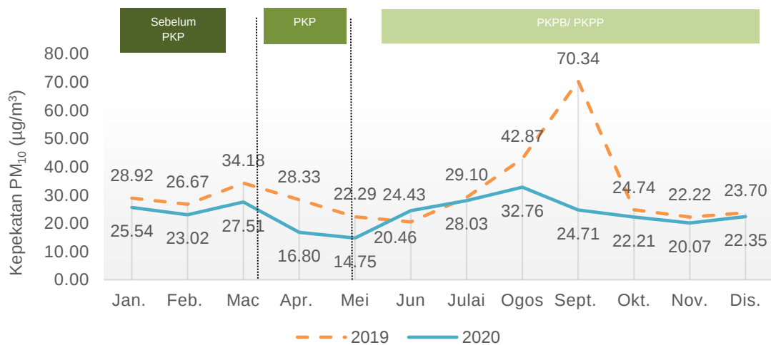
Carta 1.5: Purata bulanan kepekatan PM 10 di udara, stesen Tasek, Ipoh, Perak, 2019 dan 2020
