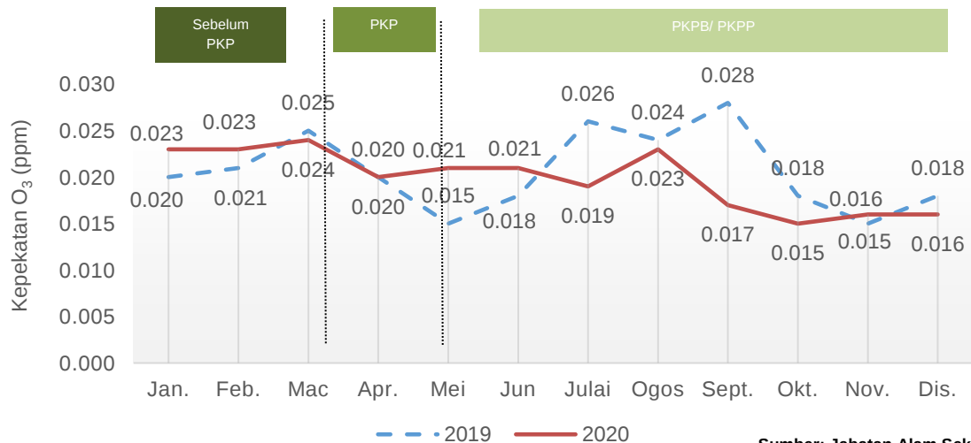
Carta 1.14: Purata bulanan kepekatan O 3 di udara, stesen Tasek, Ipoh, Perak, 2019 dan 2020
