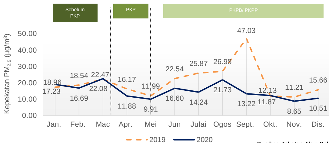
Carta 1.8: Purata bulanan kepekatan PM 2.5 di udara, stesen Taiping, Perak, 2019 dan 2020
