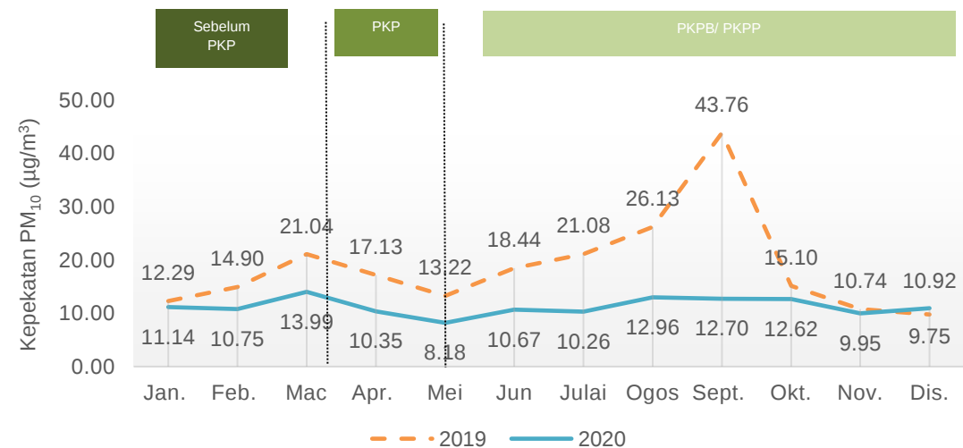
Carta 1.4: Purata bulanan kepekatan PM 10 di udara, stesen Tanjung Malim, Perak, 2019 dan 2020
