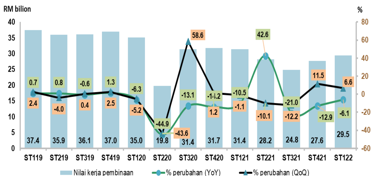
Carta 1 : Nilai kerja pembinaan dan perubahan peratus, ST1 2019 - ST1 2022
