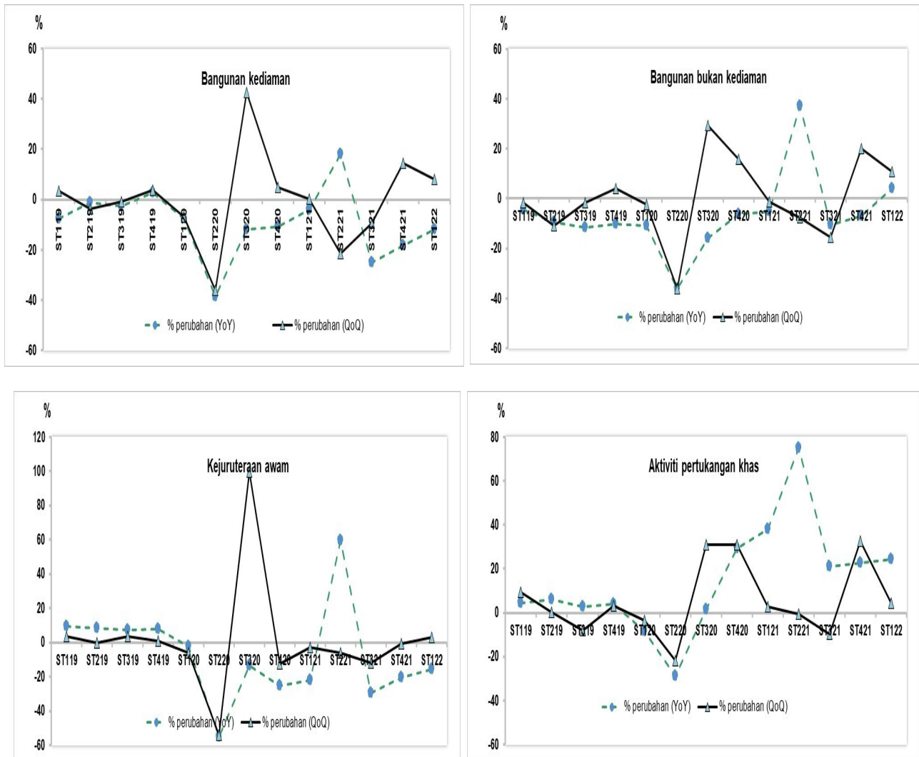
Carta 2 : Perubahan peratus tahunan mengikut subsektor, ST1 2019 - ST1 2022
